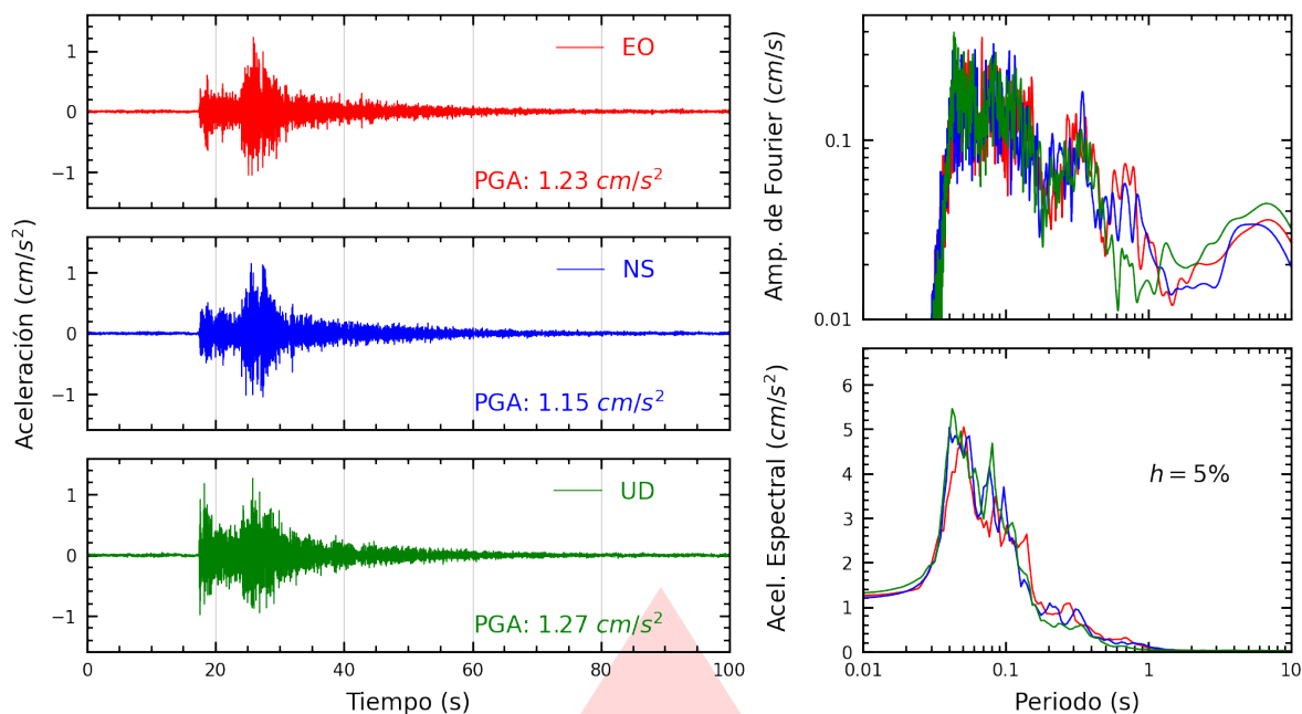
Figura A.33: Registros tiempo-historia, espectros de Fourier y de respuesta en las direcciones EO, NS y vertical de la estación UNMSM. Sismo de Callao, Provincia Constitucional del Callao del 2026-10-05, 15:24:38 (Hora local)
