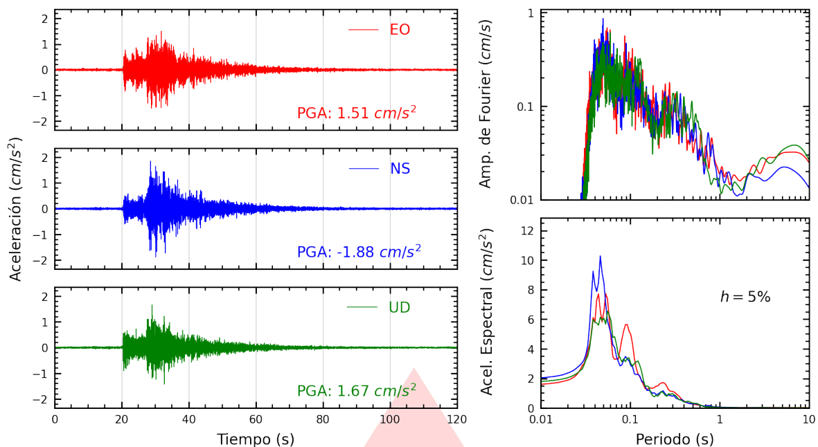
Figura A.31: Registros tiempo-historia, espectros de Fourier y de respuesta en las direcciones EO, NS y vertical de la estación IMCA. Sismo de Callao, Provincia Constitucional del Callao del 2026-10-05, 15:24:38 (Hora local)
