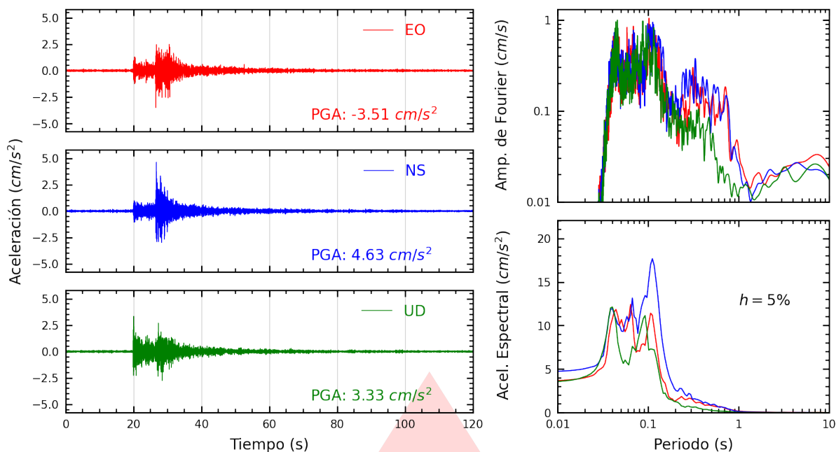
Figura A.17: Registros tiempo-historia, espectros de Fourier y de respuesta en las direcciones EO, NS y vertical de la estación MADRE. Sismo de Callao, Provincia Constitucional del Callao del 2026-10-05, 15:24:38 (Hora local)
