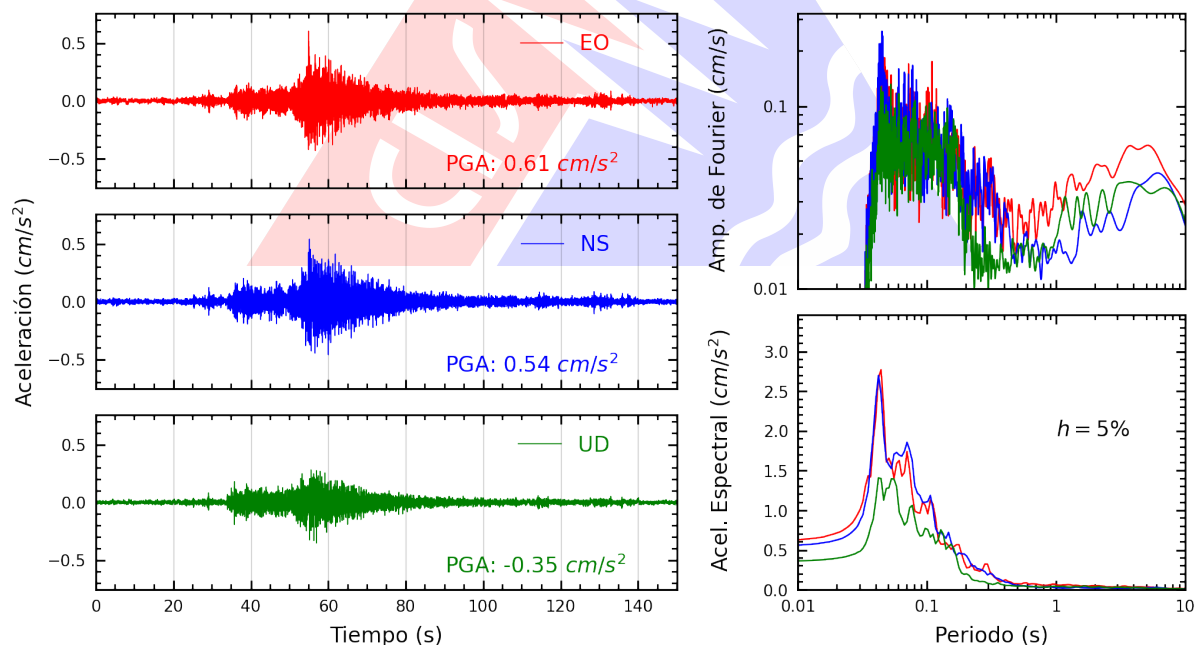
Figura A.36: Registros tiempo-historia, espectros de Fourier y de respuesta en las direcciones EO, NS y vertical de la estación UNAB. Sismo de Callao, Provincia Constitucional del Callao del 2026-10-05, 15:24:38 (Hora local)
