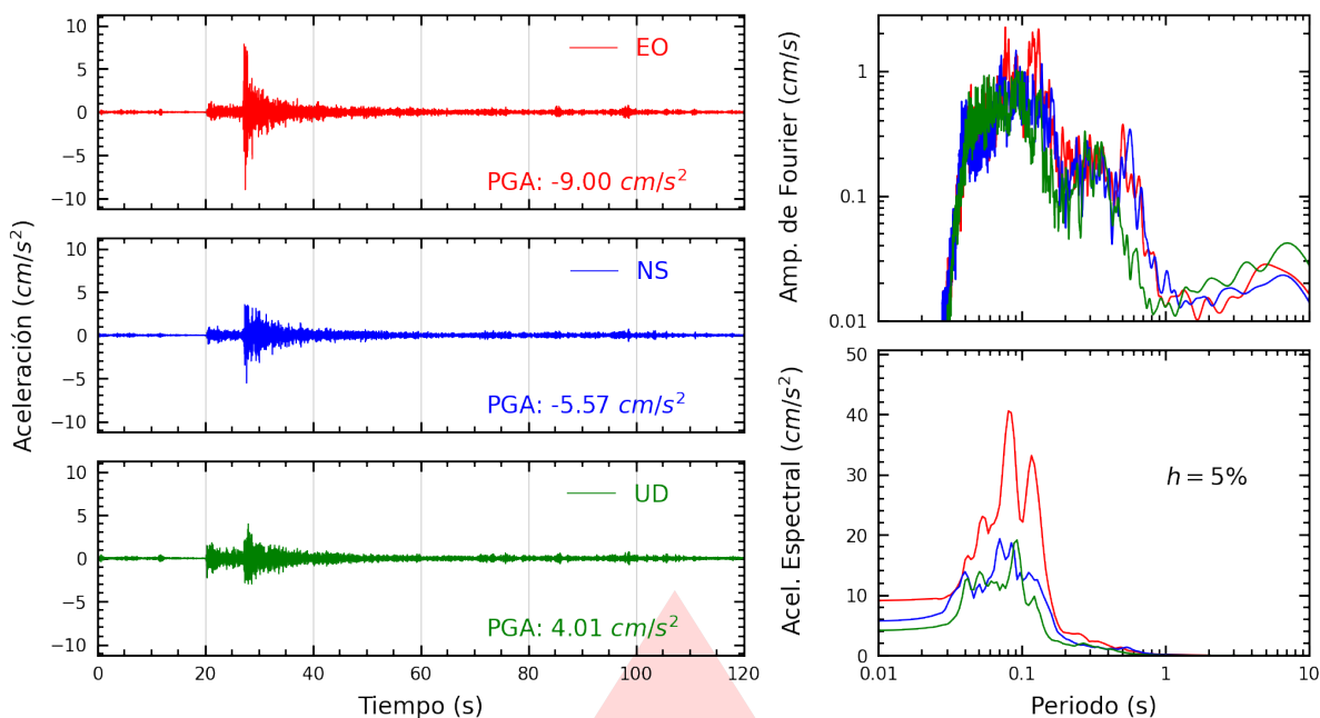
Figura A.5: Registros tiempo-historia, espectros de Fourier y de respuesta en las direcciones EO, NS y vertical de la estación SJLSV. Sismo de Callao, Provincia Constitucional del Callao del 2026-10-05, 15:24:38 (Hora local)
