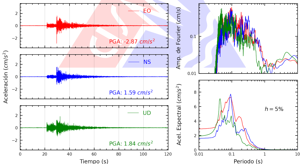
Figura A.28: Registros tiempo-historia, espectros de Fourier y de respuesta en las direcciones EO, NS y vertical de la estación USILP. Sismo de Callao, Provincia Constitucional del Callao del 2026-10-05, 15:24:38 (Hora local)
