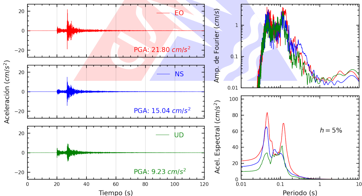
Figura A.2: Registros tiempo-historia, espectros de Fourier y de respuesta en las direcciones EO, NS y vertical de la estación AMORE. Sismo de Callao, Provincia Constitucional del Callao del 2026-10-05, 15:24:38 (Hora local)
