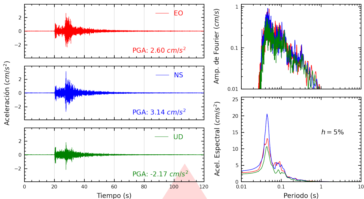
Figura A.27: Registros tiempo-historia, espectros de Fourier y de respuesta en las direcciones EO, NS y vertical de la estación BORJA. Sismo de Callao, Provincia Constitucional del Callao del 2026-10-05, 15:24:38 (Hora local)
