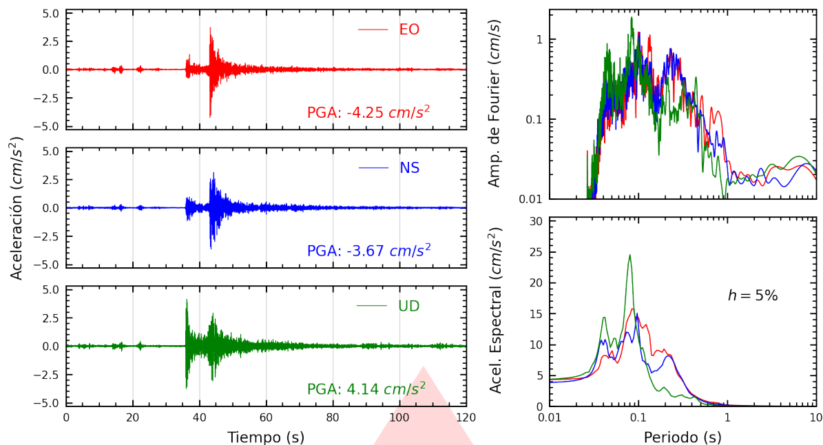
Figura A.19: Registros tiempo-historia, espectros de Fourier y de respuesta en las direcciones EO, NS y vertical de la estación SOCHO. Sismo de Callao, Provincia Constitucional del Callao del 2026-10-05, 15:24:38 (Hora local)
