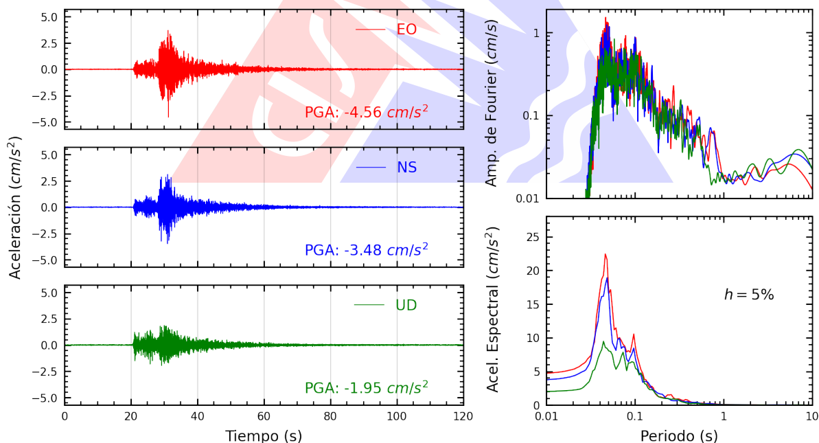
Figura A.18: Registros tiempo-historia, espectros de Fourier y de respuesta en las direcciones EO, NS y vertical de la estación UCVAT. Sismo de Callao, Provincia Constitucional del Callao del 2026-10-05, 15:24:38 (Hora local)
