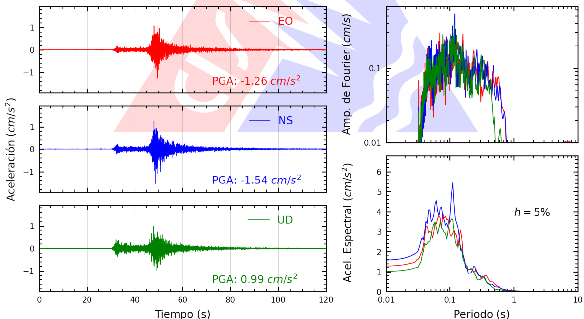
Figura A.32: Registros tiempo-historia, espectros de Fourier y de respuesta en las direcciones EO, NS y vertical de la estación CARAL. Sismo de Callao, Provincia Constitucional del Callao del 2026-10-05, 15:24:38 (Hora local)
