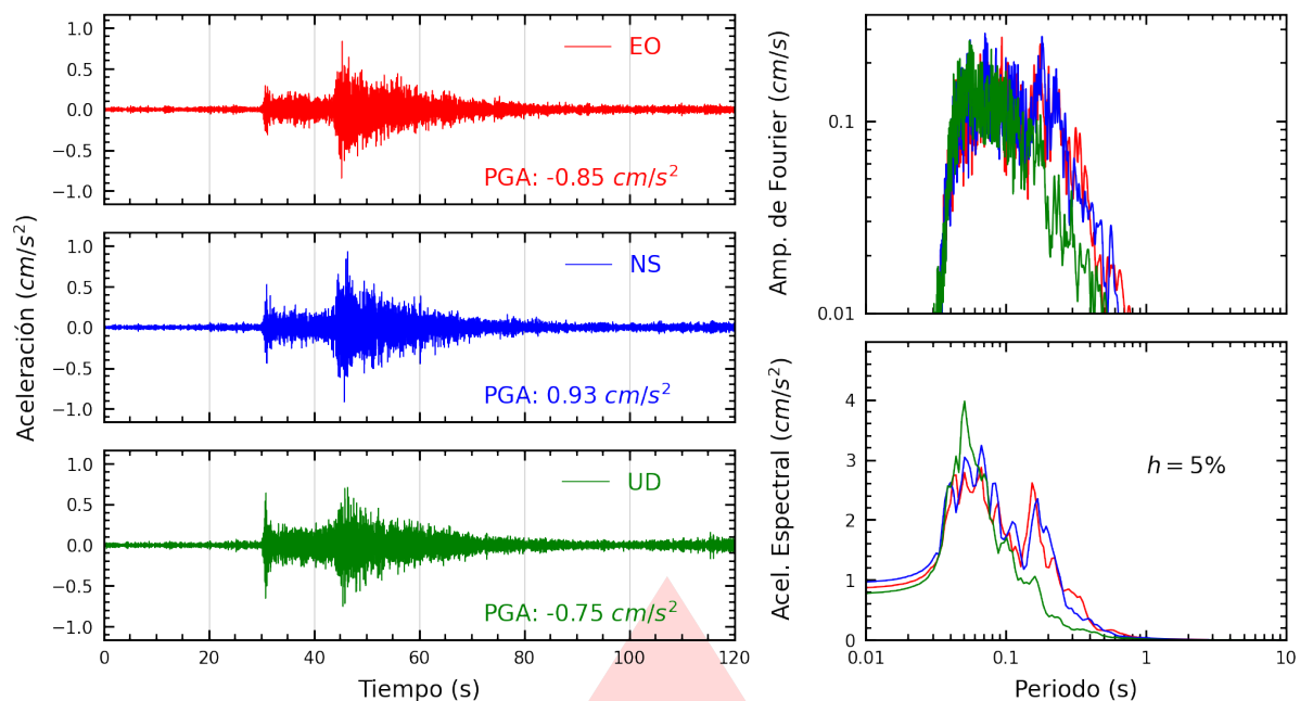
Figura A.35: Registros tiempo-historia, espectros de Fourier y de respuesta en las direcciones EO, NS y vertical de la estación ASIA. Sismo de Callao, Provincia Constitucional del Callao del 2026-10-05, 15:24:38 (Hora local)
