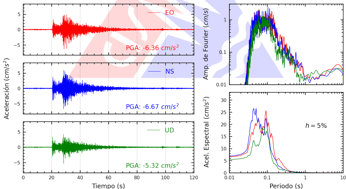
Figura A.12: Registros tiempo-historia, espectros de Fourier y de respuesta en las direcciones EO, NS y vertical de la estación USILM. Sismo de Callao, Provincia Constitucional del Callao del 2026-10-05, 15:24:38 (Hora local)
