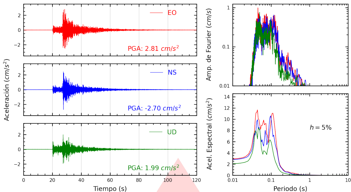
Figura A.29: Registros tiempo-historia, espectros de Fourier y de respuesta en las direcciones EO, NS y vertical de la estación ATARJ. Sismo de Callao, Provincia Constitucional del Callao del 2026-10-05, 15:24:38 (Hora local)
