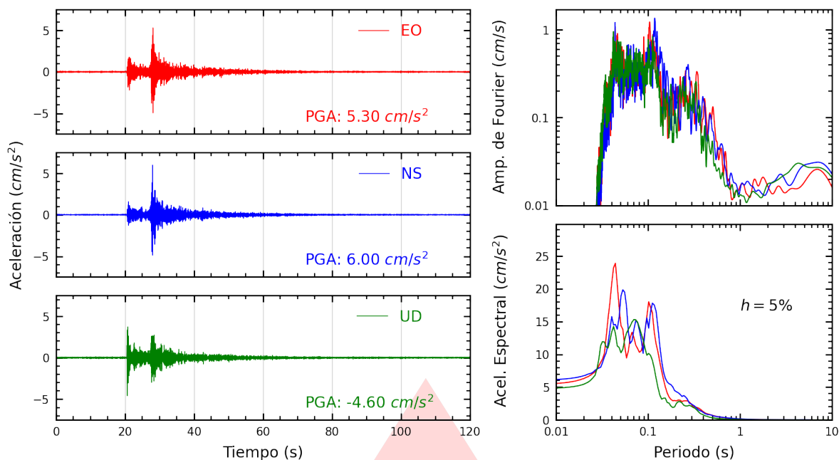
Figura A.13: Registros tiempo-historia, espectros de Fourier y de respuesta en las direcciones EO, NS y vertical de la estación URPE. Sismo de Callao, Provincia Constitucional del Callao del 2026-10-05, 15:24:38 (Hora local)
