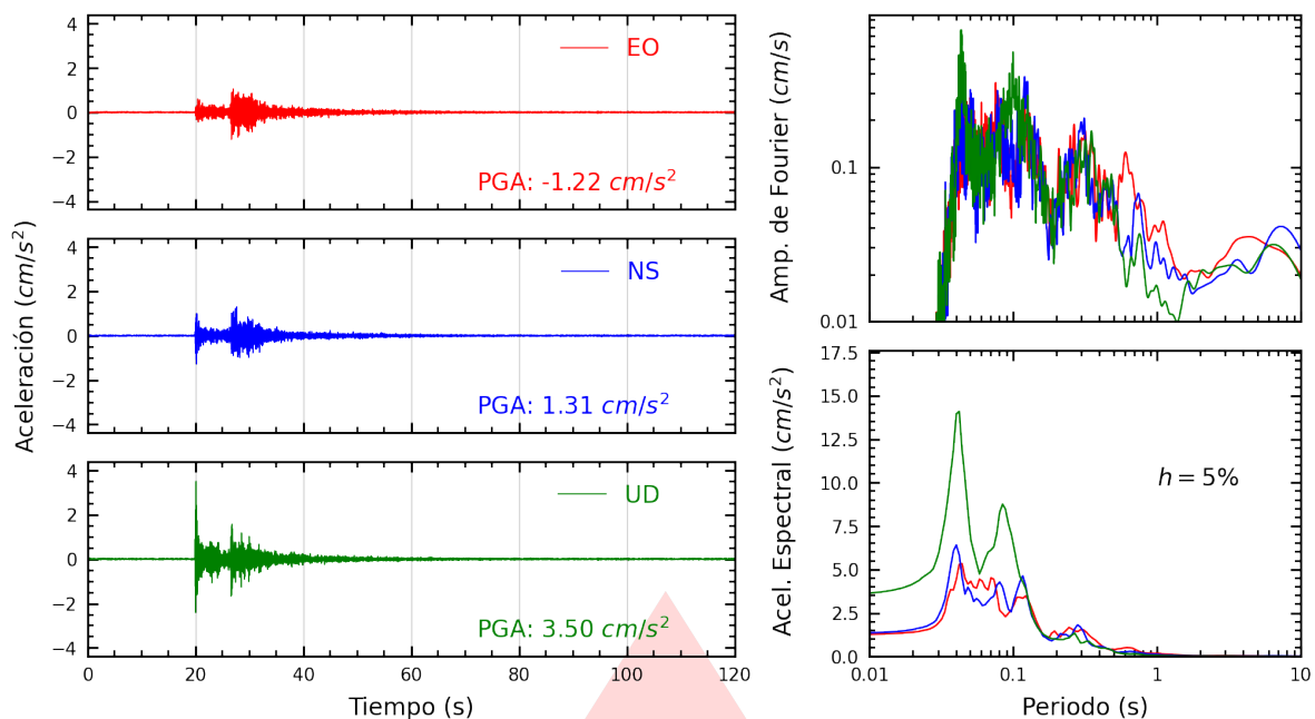
Figura A.23: Registros tiempo-historia, espectros de Fourier y de respuesta en las direcciones EO, NS y vertical de la estación BONDY. Sismo de Callao, Provincia Constitucional del Callao del 2026-10-05, 15:24:38 (Hora local)
