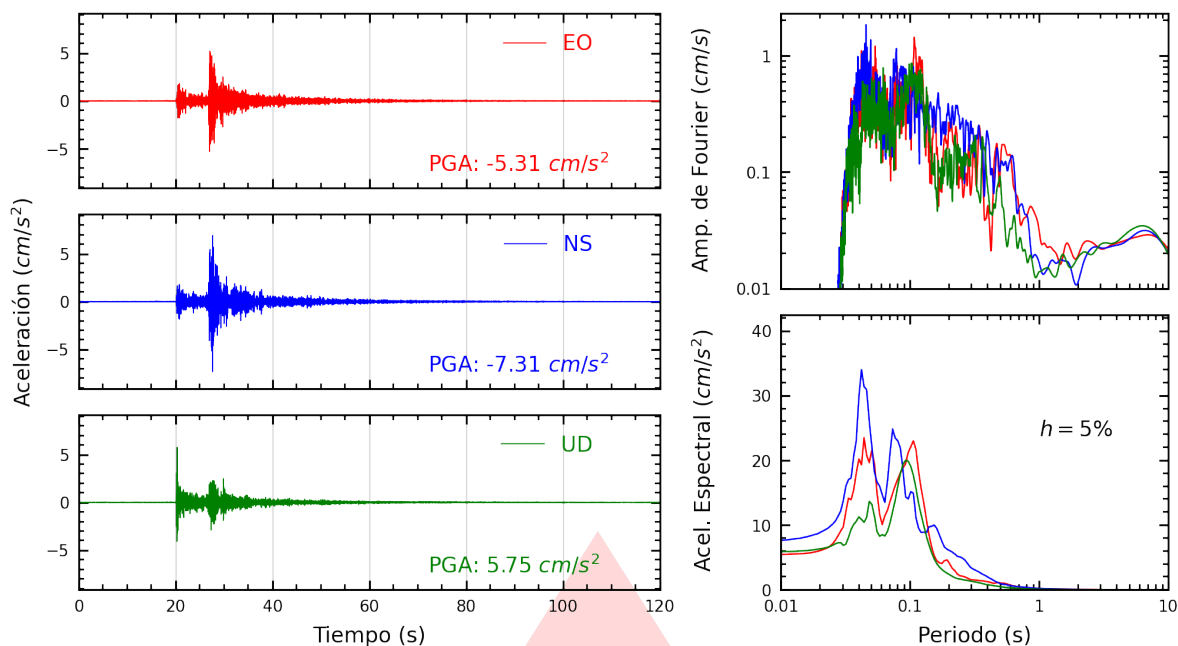
Figura A.7: Registros tiempo-historia, espectros de Fourier y de respuesta en las direcciones EO, NS y vertical de la estación COMAS. Sismo de Callao, Provincia Constitucional del Callao del 2026-10-05, 15:24:38 (Hora local)
