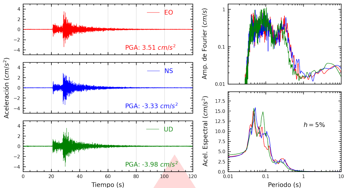
Figura A.21: Registros tiempo-historia, espectros de Fourier y de respuesta en las direcciones EO, NS y vertical de la estación SOVES. Sismo de Callao, Provincia Constitucional del Callao del 2026-10-05, 15:24:38 (Hora local)
