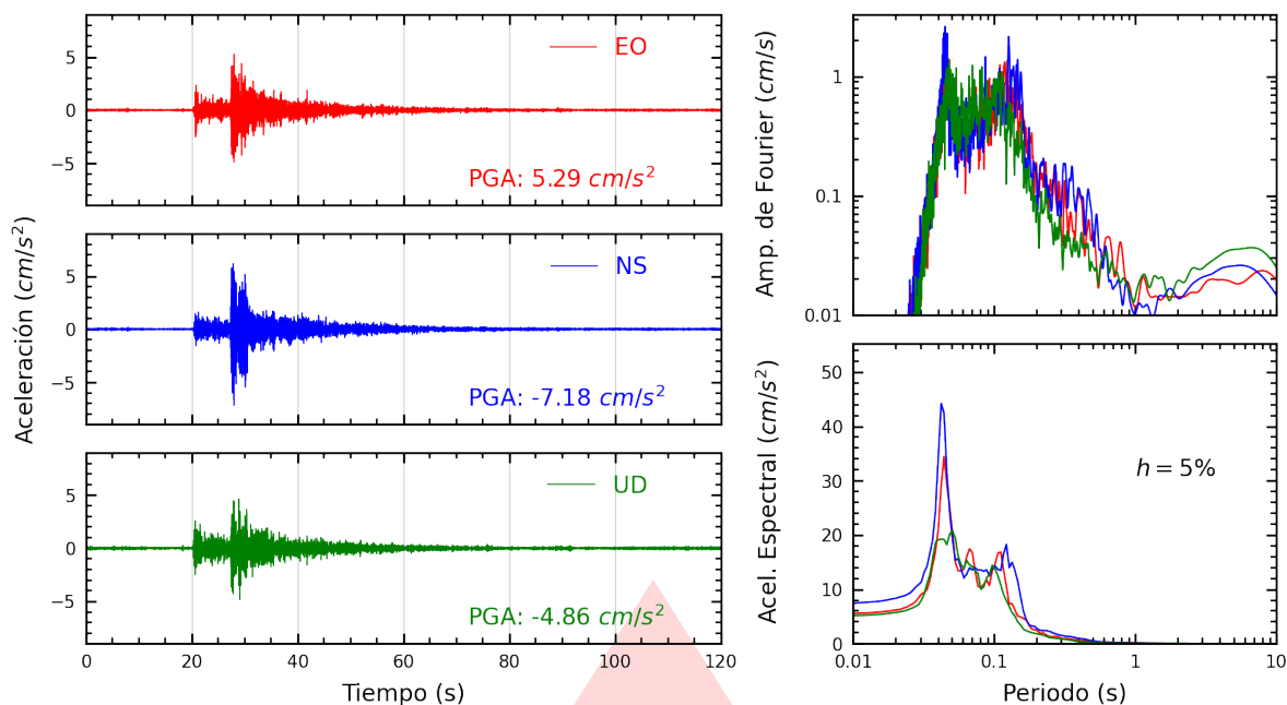
Figura A.9: Registros tiempo-historia, espectros de Fourier y de respuesta en las direcciones EO, NS y vertical de la estación CARAB. Sismo de Callao, Provincia Constitucional del Callao del 2026-10-05, 15:24:38 (Hora local)
