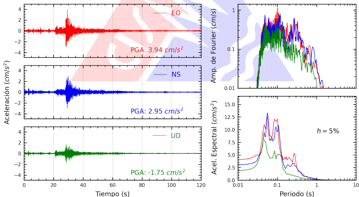
Figura A.22: Registros tiempo-historia, espectros de Fourier y de respuesta en las direcciones EO, NS y vertical de la estación BRISA. Sismo de Callao, Provincia Constitucional del Callao del 2026-10-05, 15:24:38 (Hora local)
