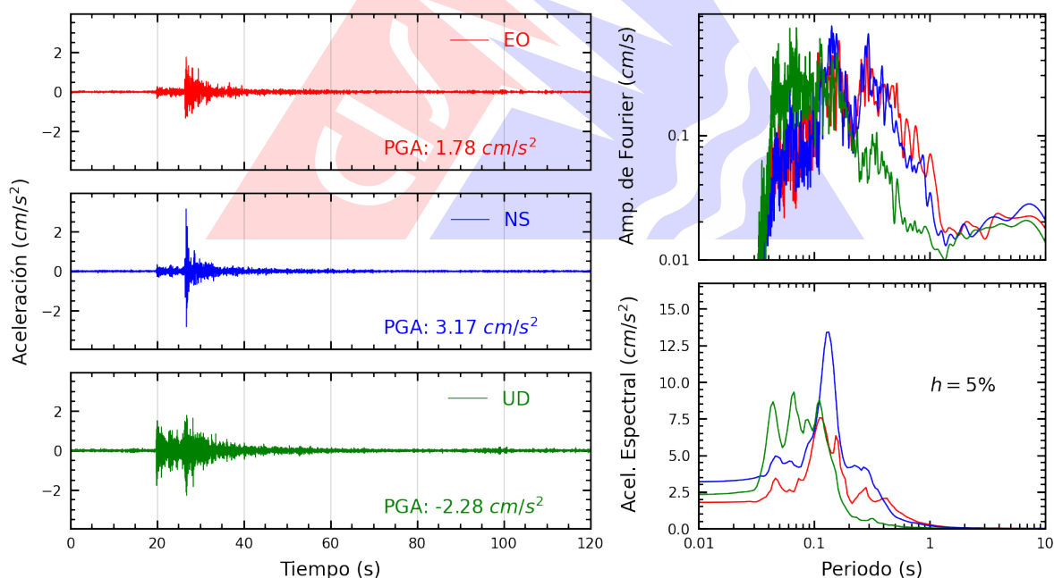
Figura A.26: Registros tiempo-historia, espectros de Fourier y de respuesta en las direcciones EO, NS y vertical de la estación ACAPU. Sismo de Callao, Provincia Constitucional del Callao del 2026-10-05, 15:24:38 (Hora local)
