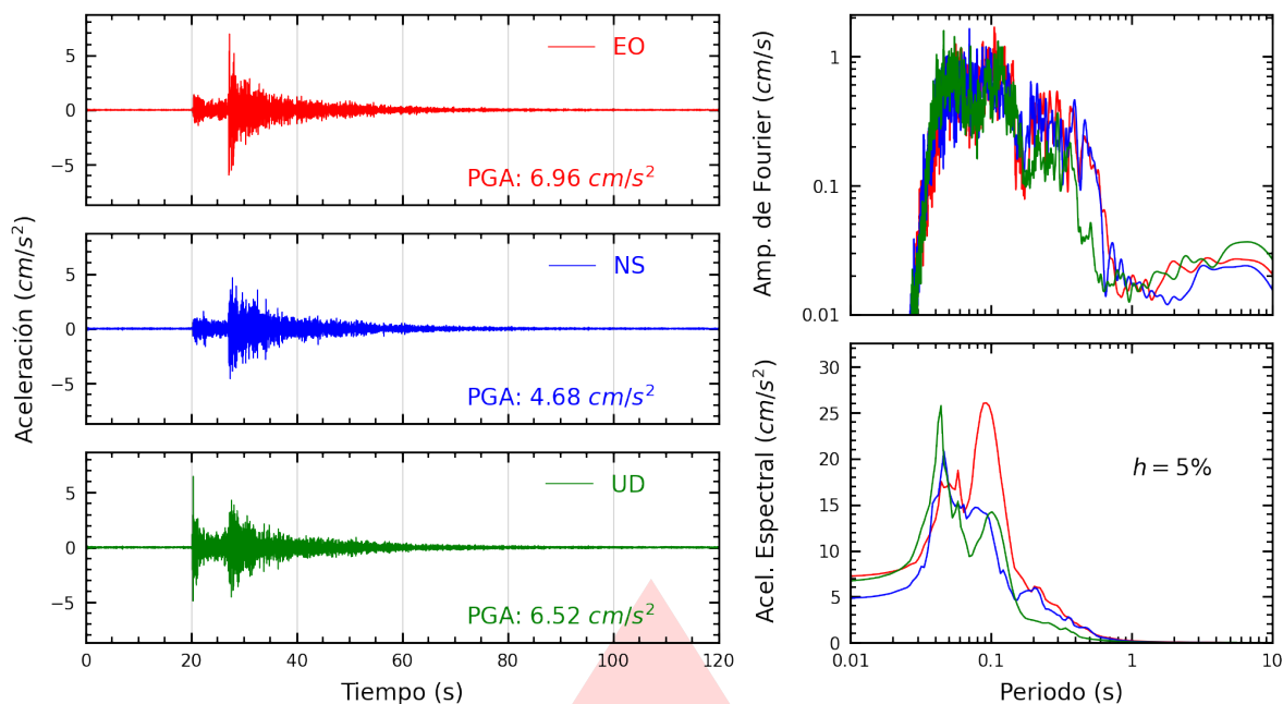
Figura A.11: Registros tiempo-historia, espectros de Fourier y de respuesta en las direcciones EO, NS y vertical de la estación SJLSC. Sismo de Callao, Provincia Constitucional del Callao del 2026-10-05, 15:24:38 (Hora local)
