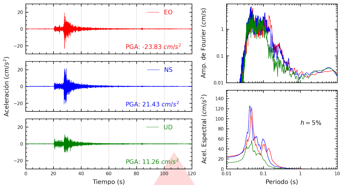
Figura A.1: Registros tiempo-historia, espectros de Fourier y de respuesta en las direcciones EO, NS y vertical de la estación SROSA. Sismo de Callao, Provincia Constitucional del Callao del 2026-10-05, 15:24:38 (Hora local)
