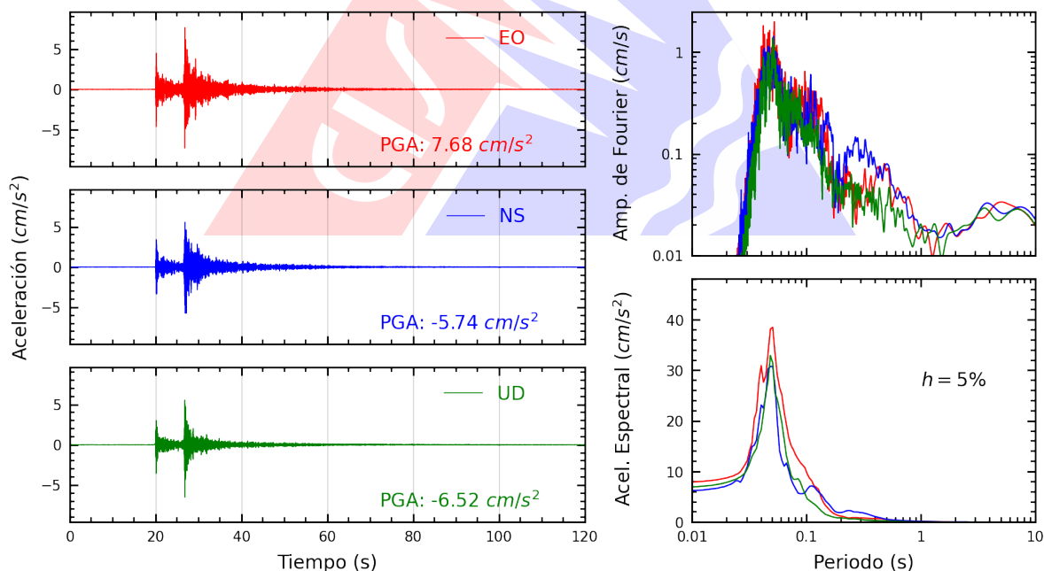
Figura A.6: Registros tiempo-historia, espectros de Fourier y de respuesta en las direcciones EO, NS y vertical de la estación UCSS. Sismo de Callao, Provincia Constitucional del Callao del 2026-10-05, 15:24:38 (Hora local)
