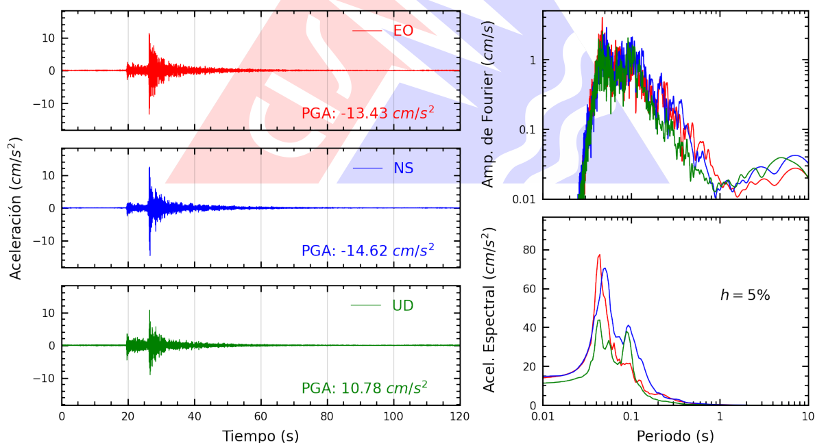
Figura A.4: Registros tiempo-historia, espectros de Fourier y de respuesta en las direcciones EO, NS y vertical de la estación INDEP. Sismo de Callao, Provincia Constitucional del Callao del 2026-10-05, 15:24:38 (Hora local)
