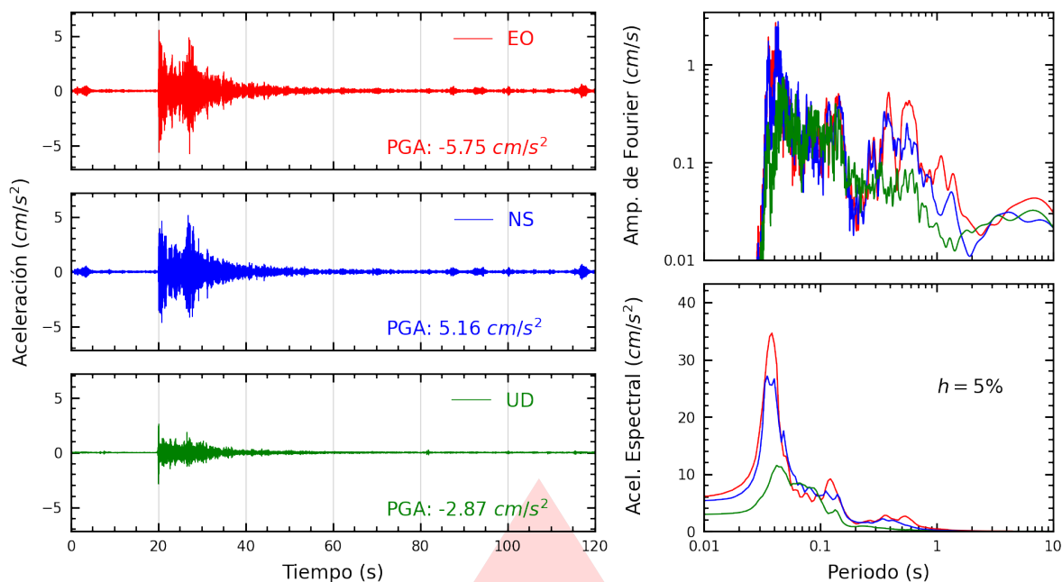
Figura A.15: Registros tiempo-historia, espectros de Fourier y de respuesta en las direcciones EO, NS y vertical de la estación DHNPE. Sismo de Callao, Provincia Constitucional del Callao del 2026-10-05, 15:24:38 (Hora local)
