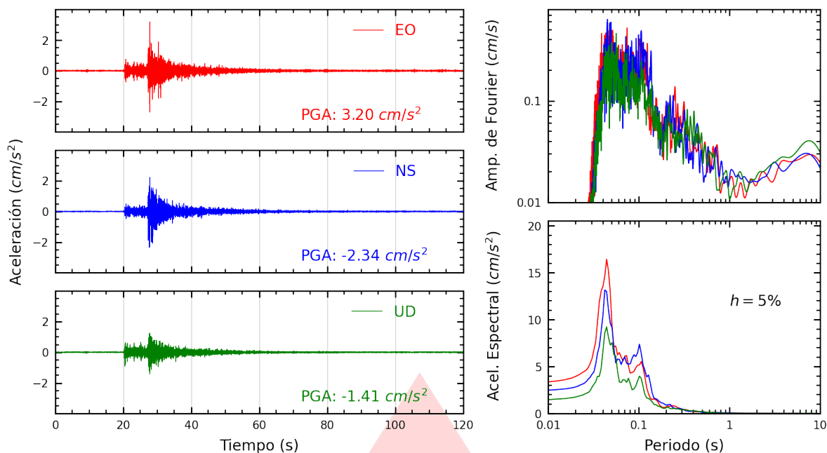
Figura A.25: Registros tiempo-historia, espectros de Fourier y de respuesta en las direcciones EO, NS y vertical de la estación INICT. Sismo de Callao, Provincia Constitucional del Callao del 2026-10-05, 15:24:38 (Hora local)
