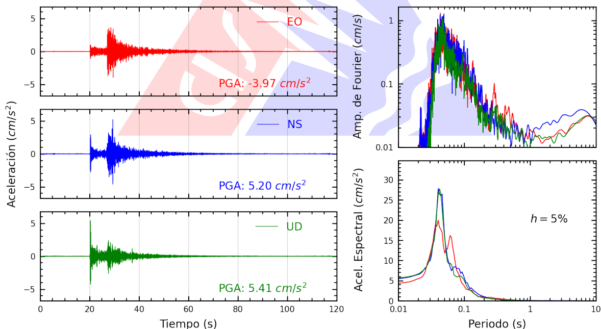
Figura A.16: Registros tiempo-historia, espectros de Fourier y de respuesta en las direcciones EO, NS y vertical de la estación SJLCE. Sismo de Callao, Provincia Constitucional del Callao del 2026-10-05, 15:24:38 (Hora local)
