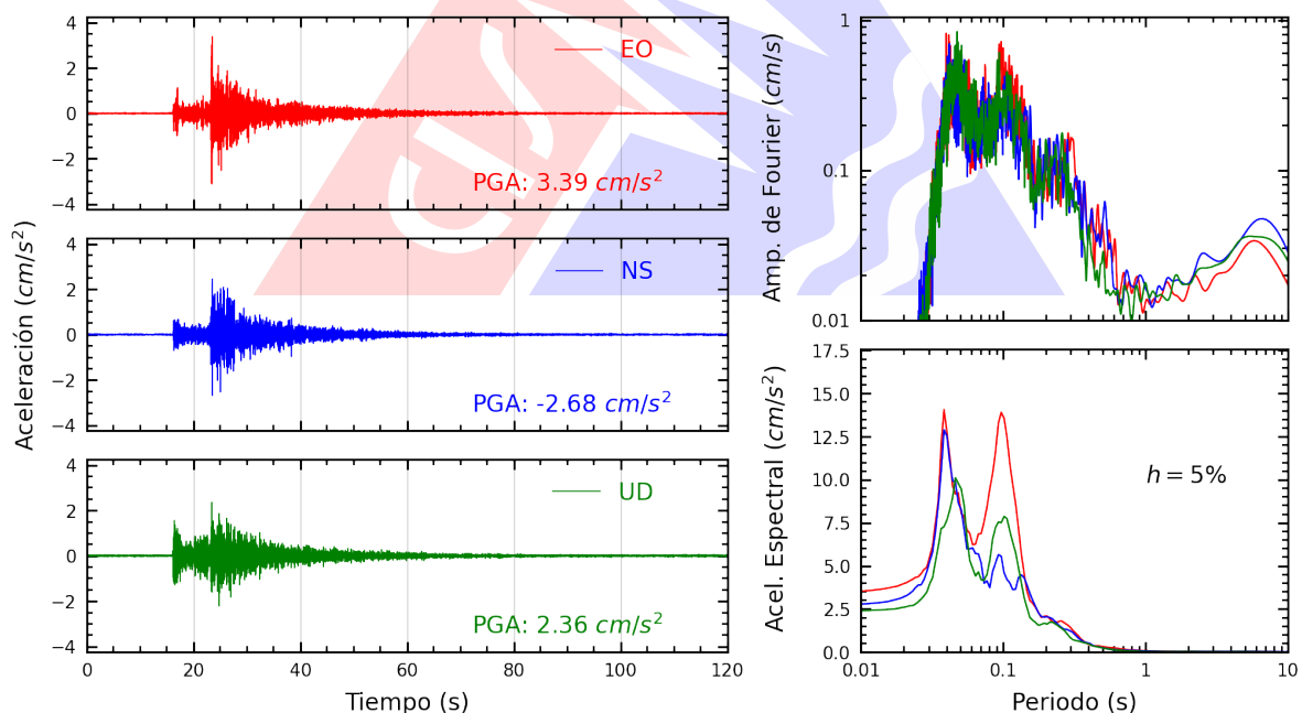
Figura A.24: Registros tiempo-historia, espectros de Fourier y de respuesta en las direcciones EO, NS y vertical de la estación USMP. Sismo de Callao, Provincia Constitucional del Callao del 2026-10-05, 15:24:38 (Hora local)
