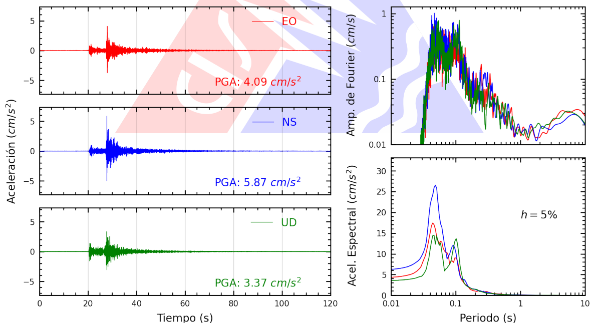
Figura A.14: Registros tiempo-historia, espectros de Fourier y de respuesta en las direcciones EO, NS y vertical de la estación SERVI. Sismo de Callao, Provincia Constitucional del Callao del 2026-10-05, 15:24:38 (Hora local)
