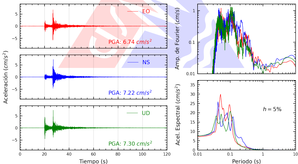
Figura A.8: Registros tiempo-historia, espectros de Fourier y de respuesta en las direcciones EO, NS y vertical de la estación JALVA. Sismo de Callao, Provincia Constitucional del Callao del 2026-10-05, 15:24:38 (Hora local)
