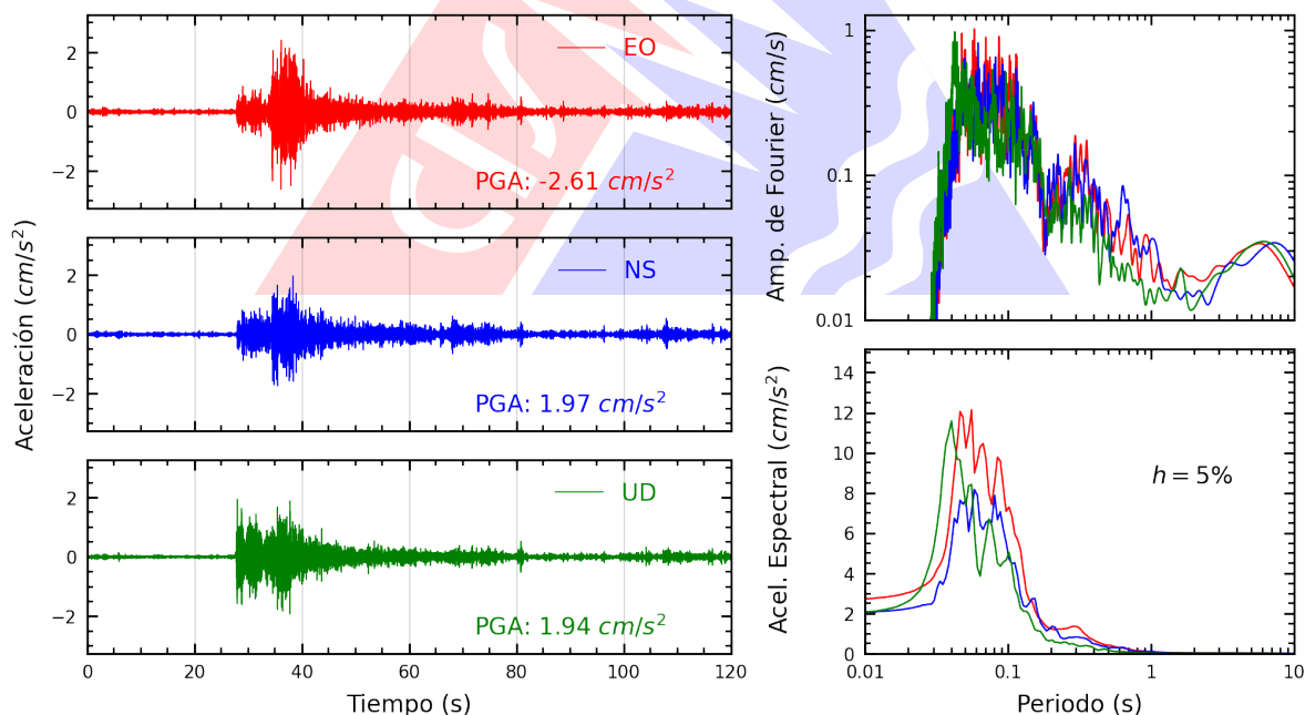
Figura A.30: Registros tiempo-historia, espectros de Fourier y de respuesta en las direcciones EO, NS y vertical de la estación UPCSM. Sismo de Callao, Provincia Constitucional del Callao del 2026-10-05, 15:24:38 (Hora local)
