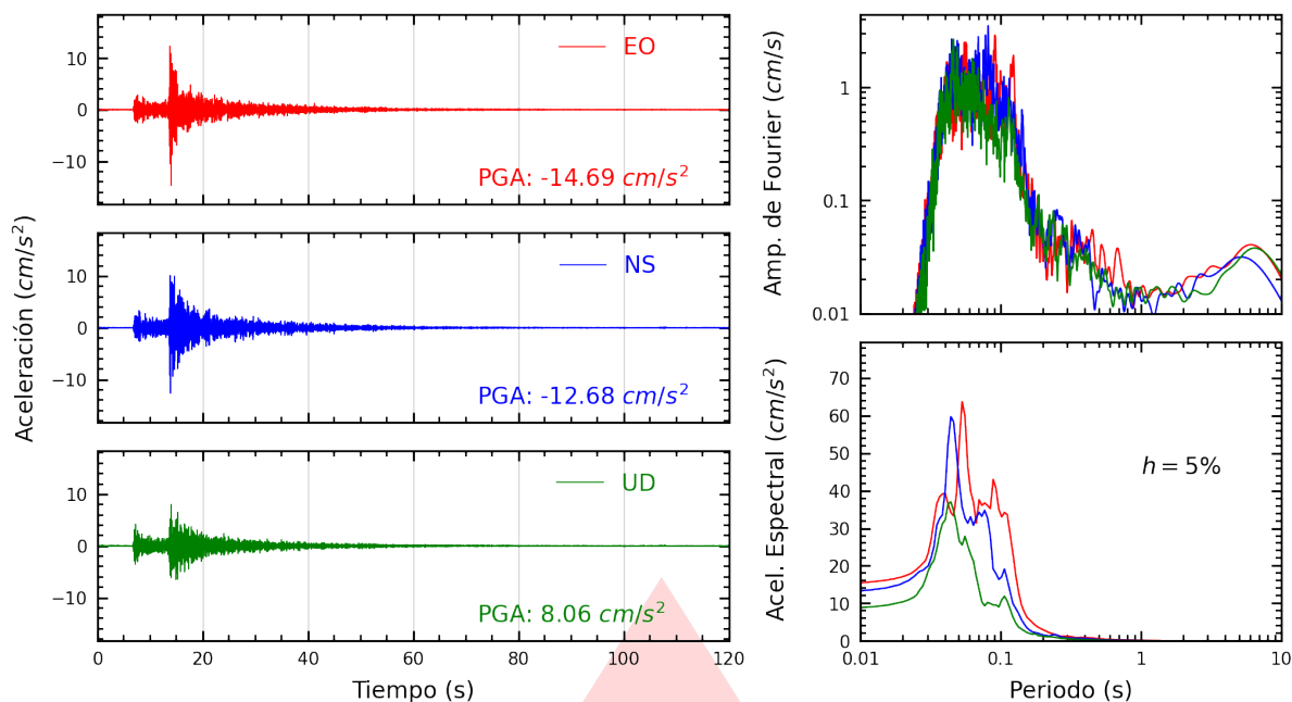
Figura A.3: Registros tiempo-historia, espectros de Fourier y de respuesta en las direcciones EO, NS y vertical de la estación JOSEO. Sismo de Callao, Provincia Constitucional del Callao del 2026-10-05, 15:24:38 (Hora local)
