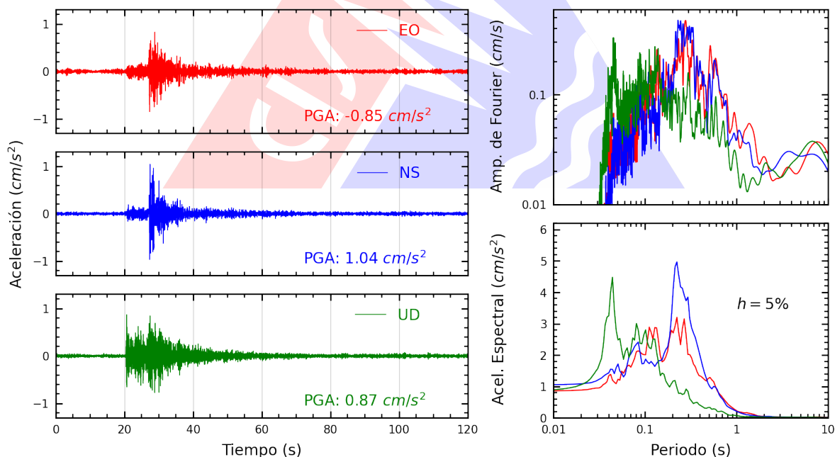
Figura A.34: Registros tiempo-historia, espectros de Fourier y de respuesta en las direcciones EO, NS y vertical de la estación DSML. Sismo de Callao, Provincia Constitucional del Callao del 2026-10-05, 15:24:38 (Hora local)
