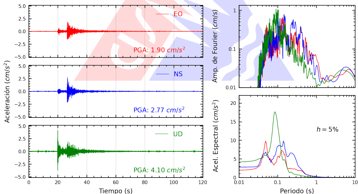
Figura A.20: Registros tiempo-historia, espectros de Fourier y de respuesta en las direcciones EO, NS y vertical de la estación RAMON. Sismo de Callao, Provincia Constitucional del Callao del 2026-10-05, 15:24:38 (Hora local)
