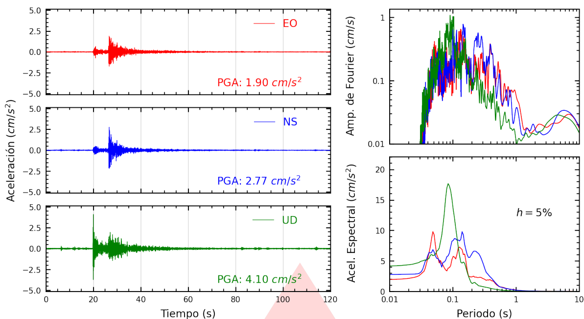
Figura A.21: Registros tiempo-historia, espectros de Fourier y de respuesta en las direcciones EO, NS y vertical de la estación RAMON. Sismo de Callao, Provincia Constitucional del Callao del 2026-10-05, 15:24:38 (Hora local)
