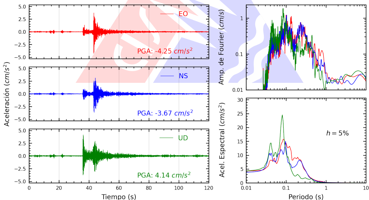
Figura A.20: Registros tiempo-historia, espectros de Fourier y de respuesta en las direcciones EO, NS y vertical de la estación SOCHO. Sismo de Callao, Provincia Constitucional del Callao del 2026-10-05, 15:24:38 (Hora local)
