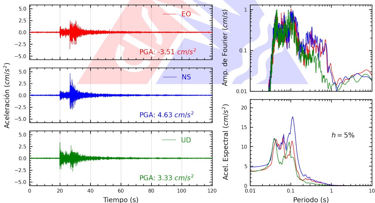
Figura A.18: Registros tiempo-historia, espectros de Fourier y de respuesta en las direcciones EO, NS y vertical de la estación MADRE. Sismo de Callao, Provincia Constitucional del Callao del 2026-10-05, 15:24:38 (Hora local)
