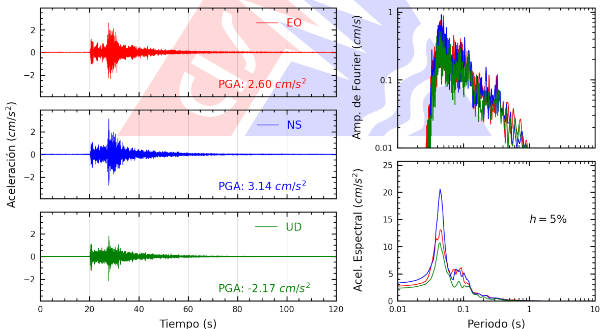
Figura A.28: Registros tiempo-historia, espectros de Fourier y de respuesta en las direcciones EO, NS y vertical de la estación BORJA. Sismo de Callao, Provincia Constitucional del Callao del 2026-10-05, 15:24:38 (Hora local)
