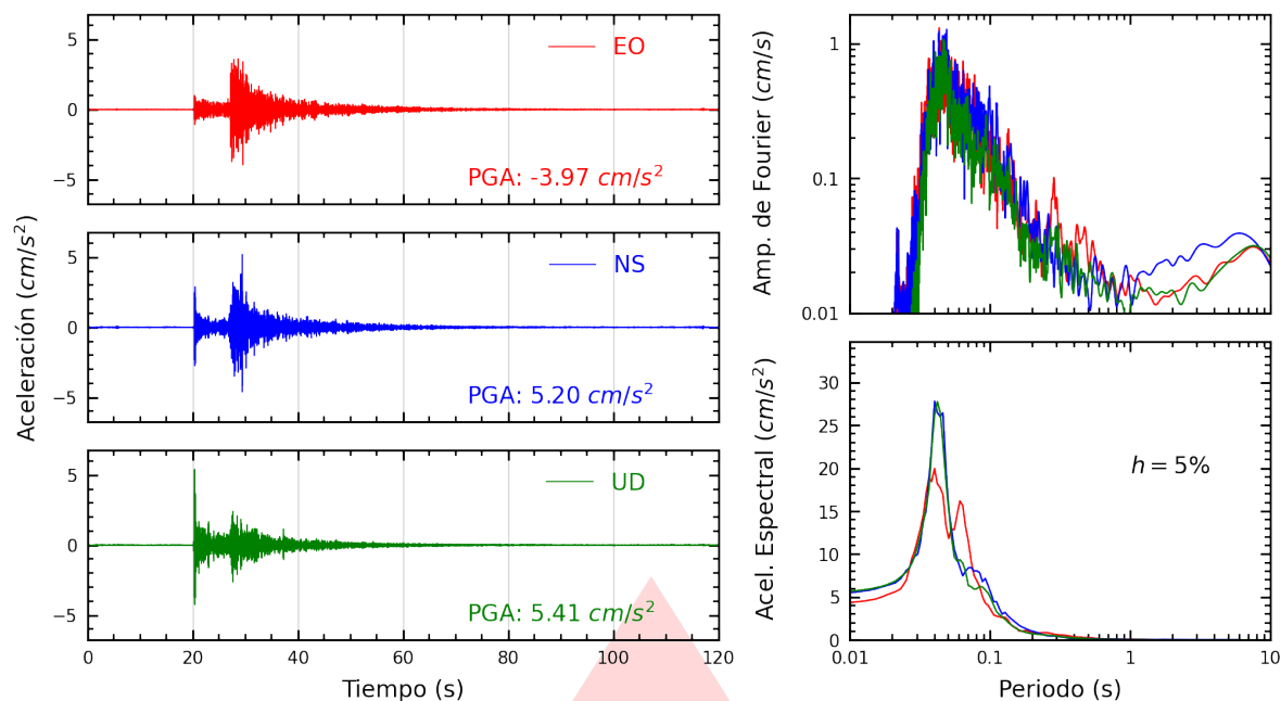
Figura A.17: Registros tiempo-historia, espectros de Fourier y de respuesta en las direcciones EO, NS y vertical de la estación SJLCE. Sismo de Callao, Provincia Constitucional del Callao del 2026-10-05, 15:24:38 (Hora local)
