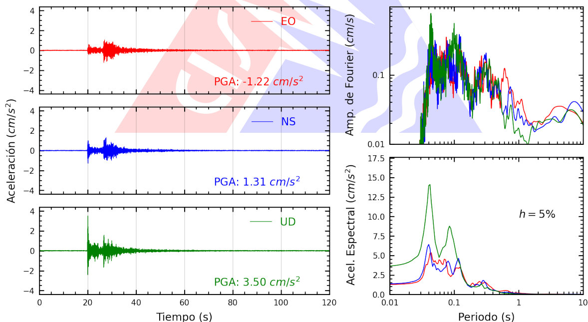
Figura A.24: Registros tiempo-historia, espectros de Fourier y de respuesta en las direcciones EO, NS y vertical de la estación BONDY. Sismo de Callao, Provincia Constitucional del Callao del 2026-10-05, 15:24:38 (Hora local)
