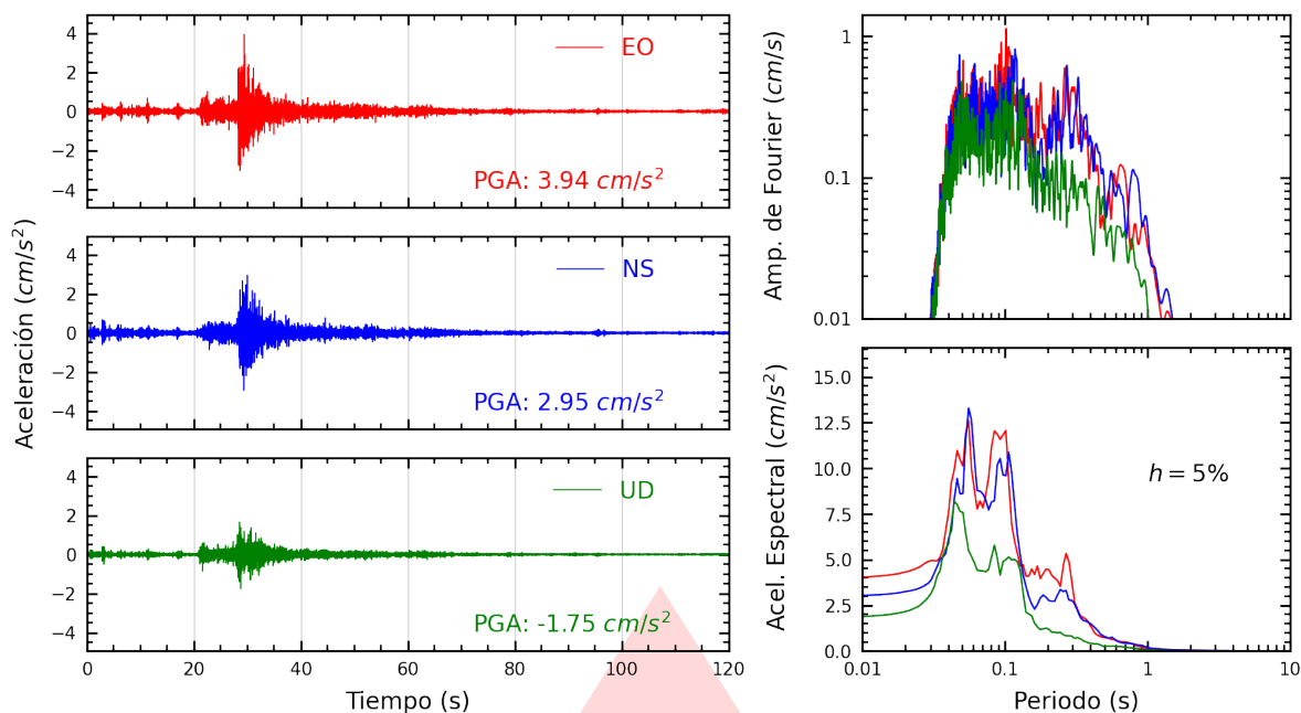
Figura A.23: Registros tiempo-historia, espectros de Fourier y de respuesta en las direcciones EO, NS y vertical de la estación BRISA. Sismo de Callao, Provincia Constitucional del Callao del 2026-10-05, 15:24:38 (Hora local)
