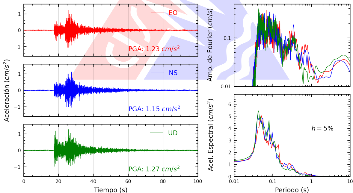
Figura A.34: Registros tiempo-historia, espectros de Fourier y de respuesta en las direcciones EO, NS y vertical de la estación UNMSM. Sismo de Callao, Provincia Constitucional del Callao del 2026-10-05, 15:24:38 (Hora local)
