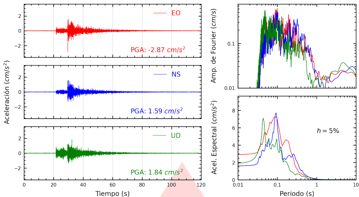
Figura A.29: Registros tiempo-historia, espectros de Fourier y de respuesta en las direcciones EO, NS y vertical de la estación USILP. Sismo de Callao, Provincia Constitucional del Callao del 2026-10-05, 15:24:38 (Hora local)
