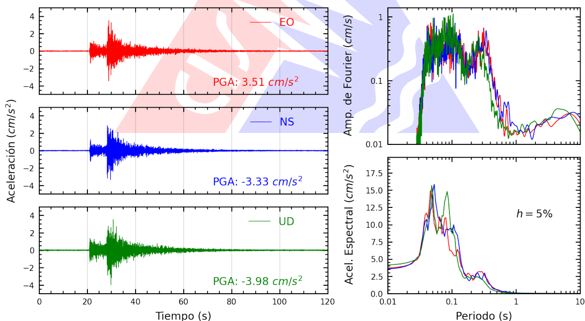
Figura A.22: Registros tiempo-historia, espectros de Fourier y de respuesta en las direcciones EO, NS y vertical de la estación SOVES. Sismo de Callao, Provincia Constitucional del Callao del 2026-10-05, 15:24:38 (Hora local)
