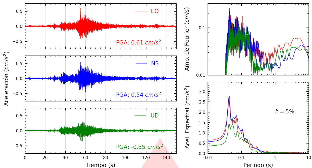
Figura A.37: Registros tiempo-historia, espectros de Fourier y de respuesta en las direcciones EO, NS y vertical de la estación UNAB. Sismo de Callao, Provincia Constitucional del Callao del 2026-10-05, 15:24:38 (Hora local)
