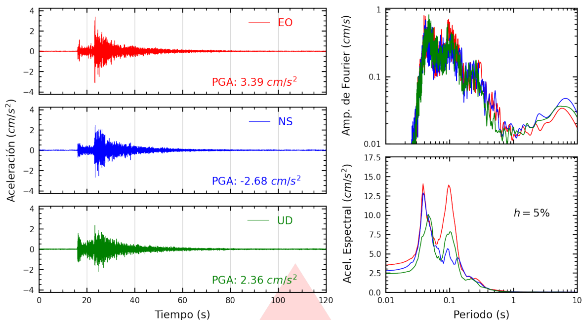
Figura A.25: Registros tiempo-historia, espectros de Fourier y de respuesta en las direcciones EO, NS y vertical de la estación USMP. Sismo de Callao, Provincia Constitucional del Callao del 2026-10-05, 15:24:38 (Hora local)
