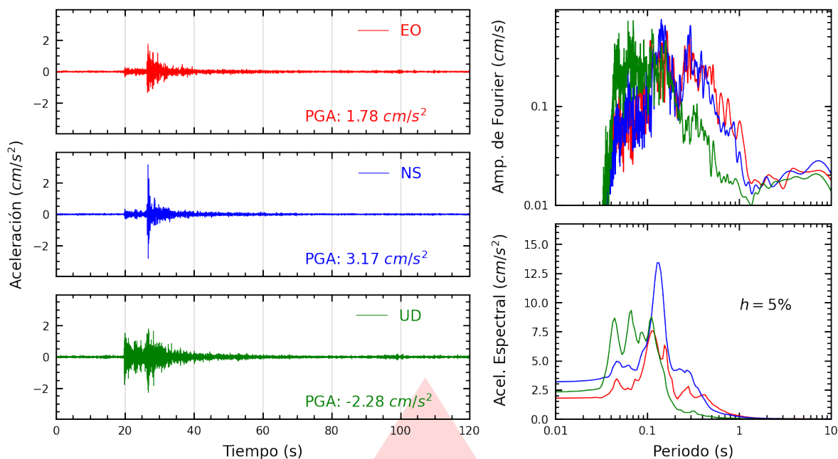
Figura A.27: Registros tiempo-historia, espectros de Fourier y de respuesta en las direcciones EO, NS y vertical de la estación ACAPU. Sismo de Callao, Provincia Constitucional del Callao del 2026-10-05, 15:24:38 (Hora local)
