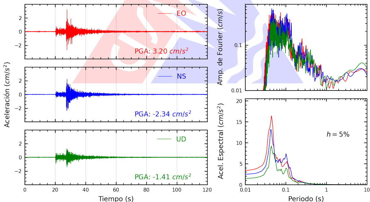
Figura A.26: Registros tiempo-historia, espectros de Fourier y de respuesta en las direcciones EO, NS y vertical de la estación INICT. Sismo de Callao, Provincia Constitucional del Callao del 2026-10-05, 15:24:38 (Hora local)
