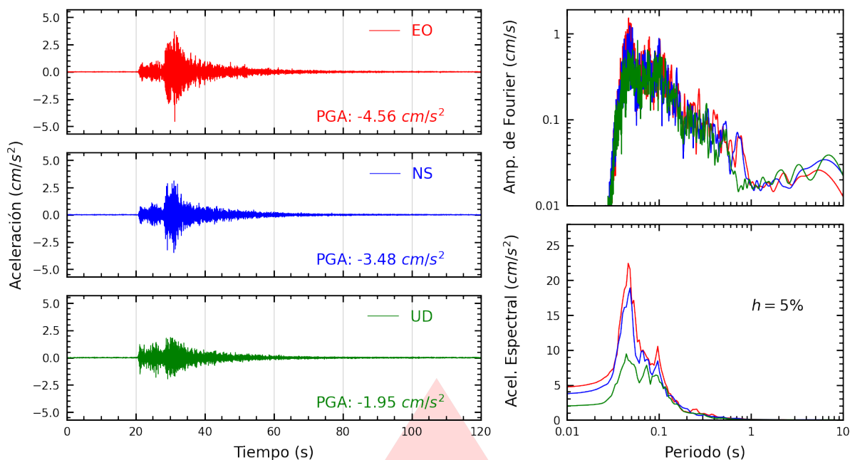
Figura A.19: Registros tiempo-historia, espectros de Fourier y de respuesta en las direcciones EO, NS y vertical de la estación UCVAT. Sismo de Callao, Provincia Constitucional del Callao del 2026-10-05, 15:24:38 (Hora local)
