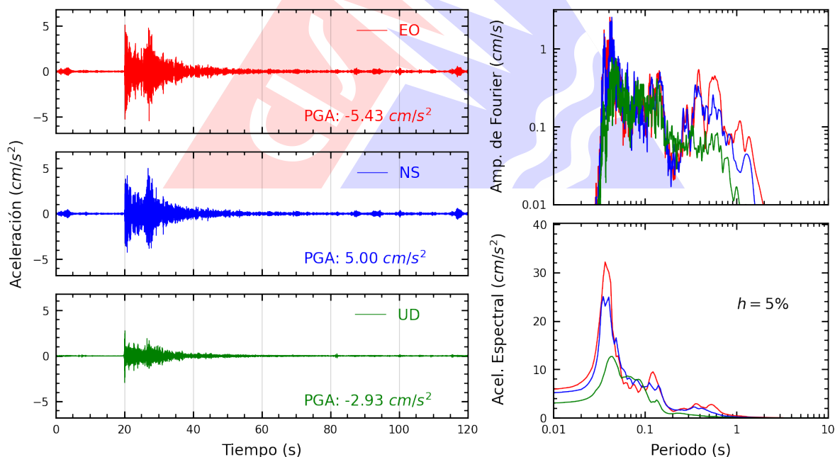
Figura A.16: Registros tiempo-historia, espectros de Fourier y de respuesta en las direcciones EO, NS y vertical de la estación DHN2. Sismo de Callao, Provincia Constitucional del Callao del 2026-10-05, 15:24:38 (Hora local)
