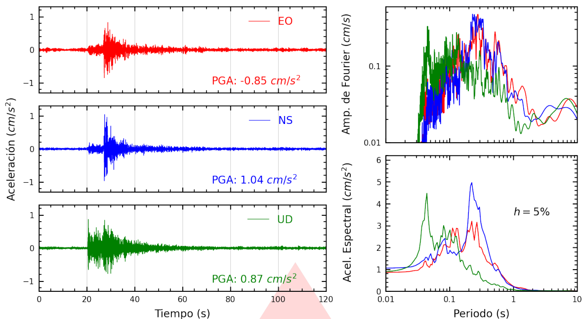
Figura A.35: Registros tiempo-historia, espectros de Fourier y de respuesta en las direcciones EO, NS y vertical de la estación DSML. Sismo de Callao, Provincia Constitucional del Callao del 2026-10-05, 15:24:38 (Hora local)
