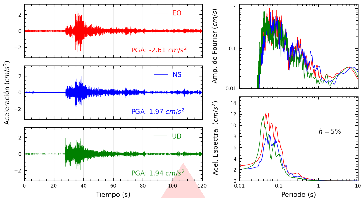
Figura A.31: Registros tiempo-historia, espectros de Fourier y de respuesta en las direcciones EO, NS y vertical de la estación UPCSM. Sismo de Callao, Provincia Constitucional del Callao del 2026-10-05, 15:24:38 (Hora local)
