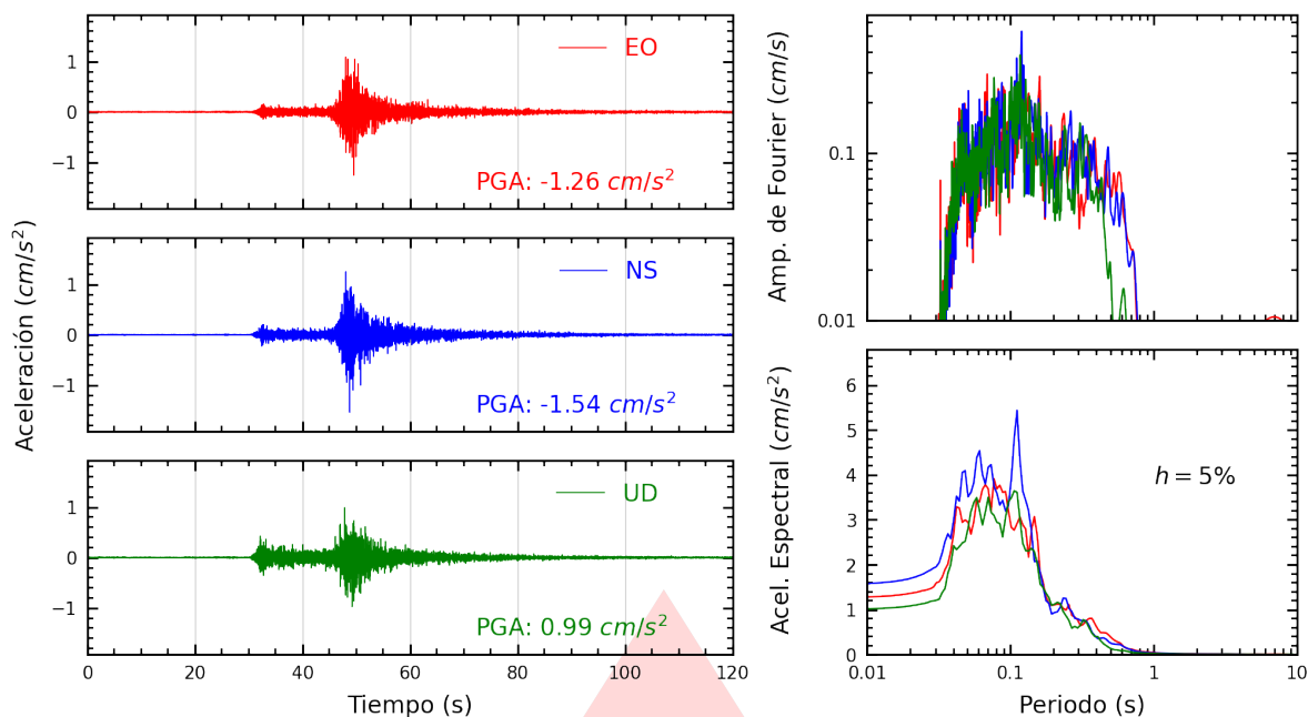
Figura A.33: Registros tiempo-historia, espectros de Fourier y de respuesta en las direcciones EO, NS y vertical de la estación CARAL. Sismo de Callao, Provincia Constitucional del Callao del 2026-10-05, 15:24:38 (Hora local)
