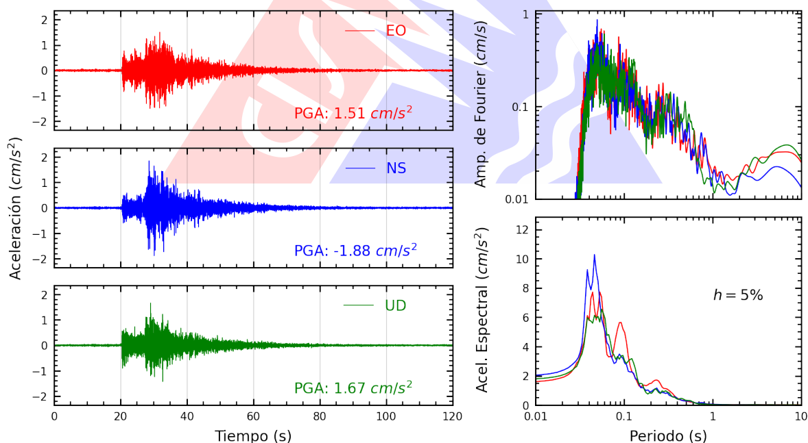
Figura A.32: Registros tiempo-historia, espectros de Fourier y de respuesta en las direcciones EO, NS y vertical de la estación IMCA. Sismo de Callao, Provincia Constitucional del Callao del 2026-10-05, 15:24:38 (Hora local)
