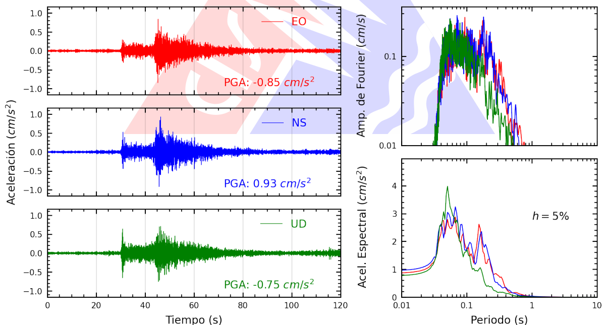
Figura A.36: Registros tiempo-historia, espectros de Fourier y de respuesta en las direcciones EO, NS y vertical de la estación ASIA. Sismo de Callao, Provincia Constitucional del Callao del 2026-10-05, 15:24:38 (Hora local)
