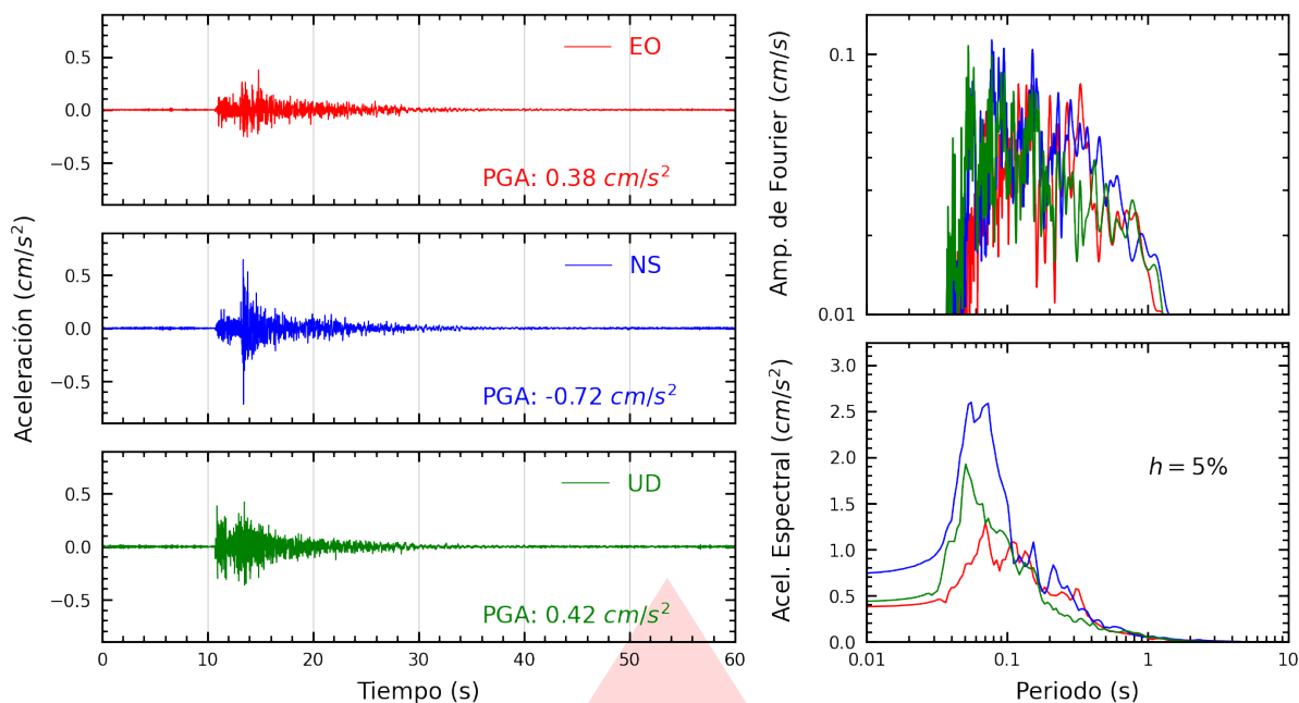
Figura A.1: Registros tiempo-historia, espectros de Fourier y de respuesta en las direcciones EO, NS y vertical de la estación SCHYO. Sismo de Chupaca, Chupaca - Junín del 2026-10-06, 23:43:06 (Hora local)
