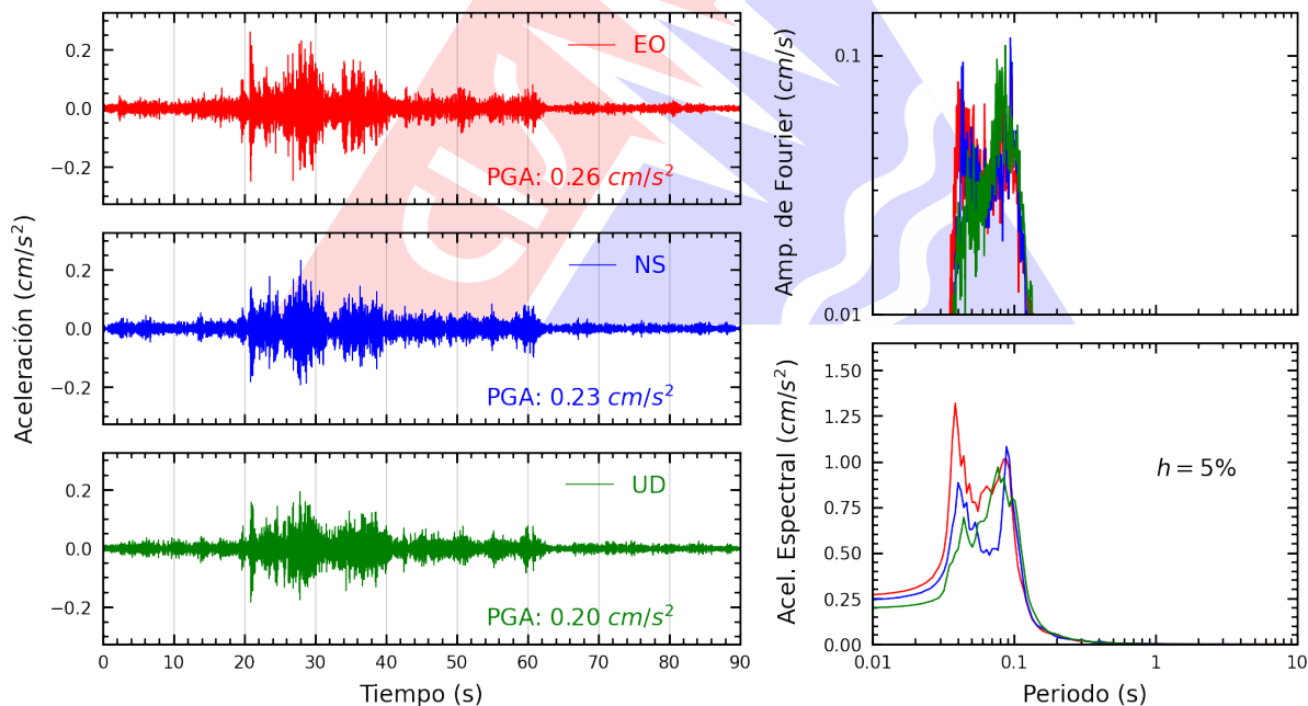
Figura A.2: Registros tiempo-historia, espectros de Fourier y de respuesta en las direcciones EO, NS y vertical de la estación SCAYA. Sismo de Chupaca, Chupaca - Junín del 2026-10-06, 23:43:06 (Hora local)
