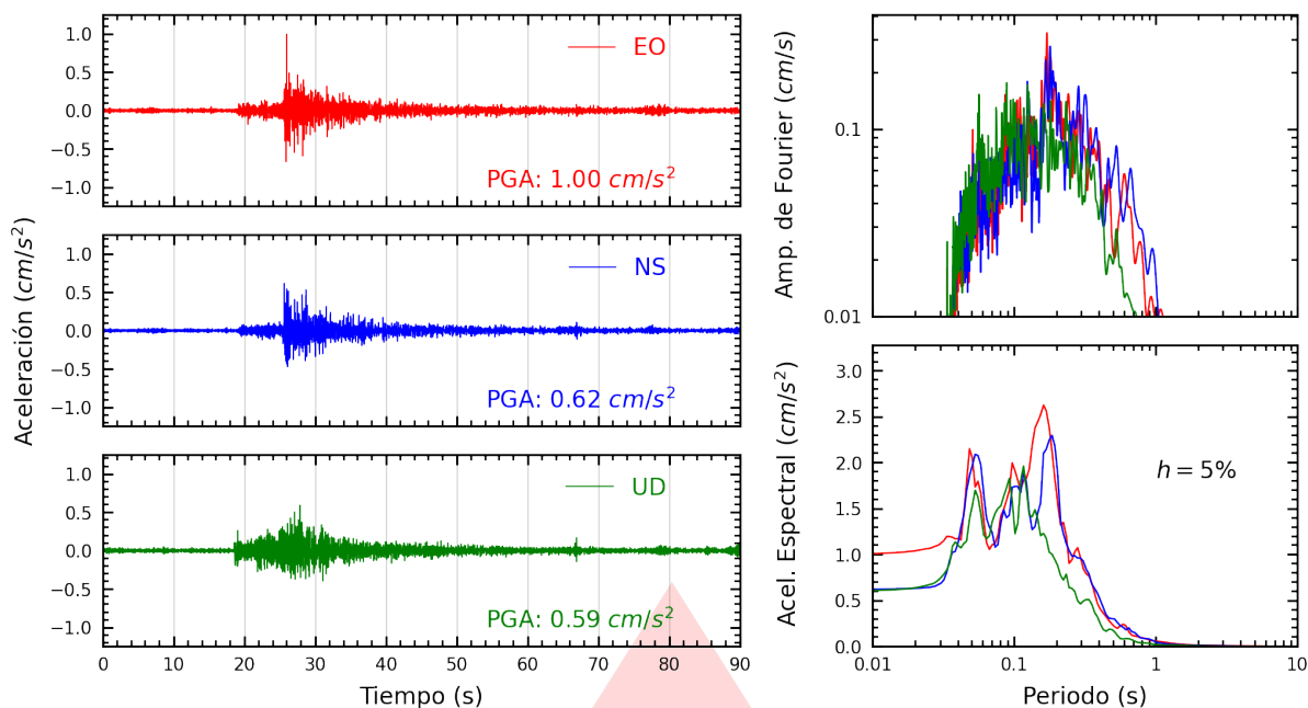
Figura A.1: Registros tiempo-historia, espectros de Fourier y de respuesta en las direcciones EO, NS y vertical de la estación SCICA. Sismo de Ica, Ica - Ica del 2026-10-07, 01:16:38 (Hora local)
