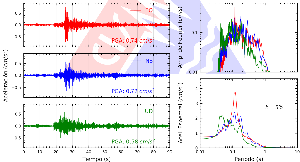
Figura A.2: Registros tiempo-historia, espectros de Fourier y de respuesta en las direcciones EO, NS y vertical de la estación UNICA. Sismo de Ica, Ica - Ica del 2026-10-07, 01:16:38 (Hora local)
