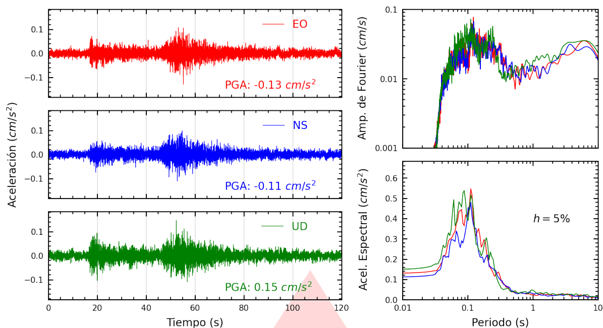
Figura A.3: Registros tiempo-historia, espectros de Fourier y de respuesta en las direcciones EO, NS y vertical de la estación SOVES. Sismo de Ica, Ica - Ica del 2026-10-07, 01:16:38 (Hora local)
