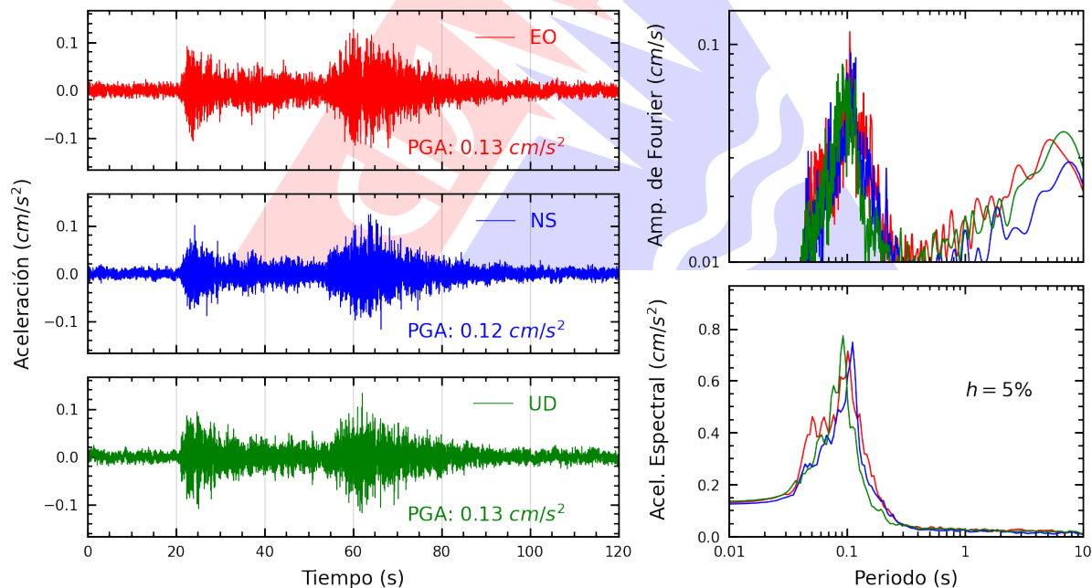
Figura A.4: Registros tiempo-historia, espectros de Fourier y de respuesta en las direcciones EO, NS y vertical de la estación AMORE. Sismo de Ica, Ica - Ica del 2026-10-07, 01:16:38 (Hora local)
