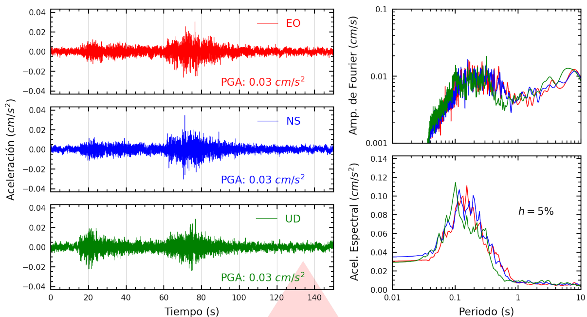
Figura A.5: Registros tiempo-historia, espectros de Fourier y de respuesta en las direcciones EO, NS y vertical de la estación CARAL. Sismo de Ica, Ica - Ica del 2026-10-07, 01:16:38 (Hora local)
