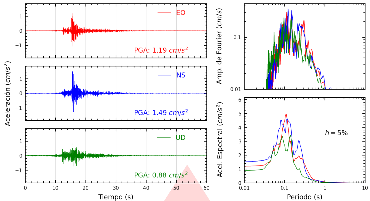
Figura A.1: Registros tiempo-historia, espectros de Fourier y de respuesta en las direcciones EO, NS y vertical de la estación SCHYO. Sismo de Chupaca, Chupaca - Junín del 2026-10-07, 03:42:38 (Hora local)
