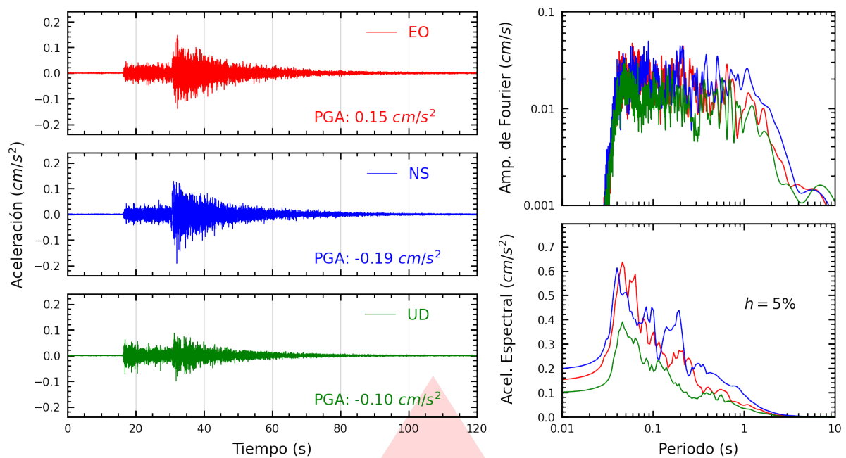
Figura A.1: Registros tiempo-historia, espectros de Fourier y de respuesta en las direcciones EO, NS y vertical de la estación UNSA2. Sismo de Aplao, Castilla - Arequipa del 2026-10-09, 05:55:25 (Hora local)
