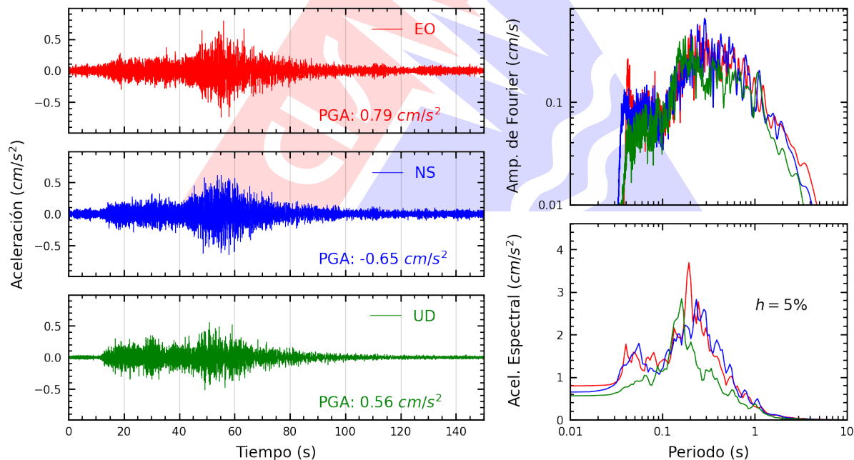
Figura A.4: Registros tiempo-historia, espectros de Fourier y de respuesta en las direcciones EO, NS y vertical de la estación UPTAC. Sismo de Quilca, Camaná - Arequipa del 2026-10-11, 08:43:01 (Hora local)
