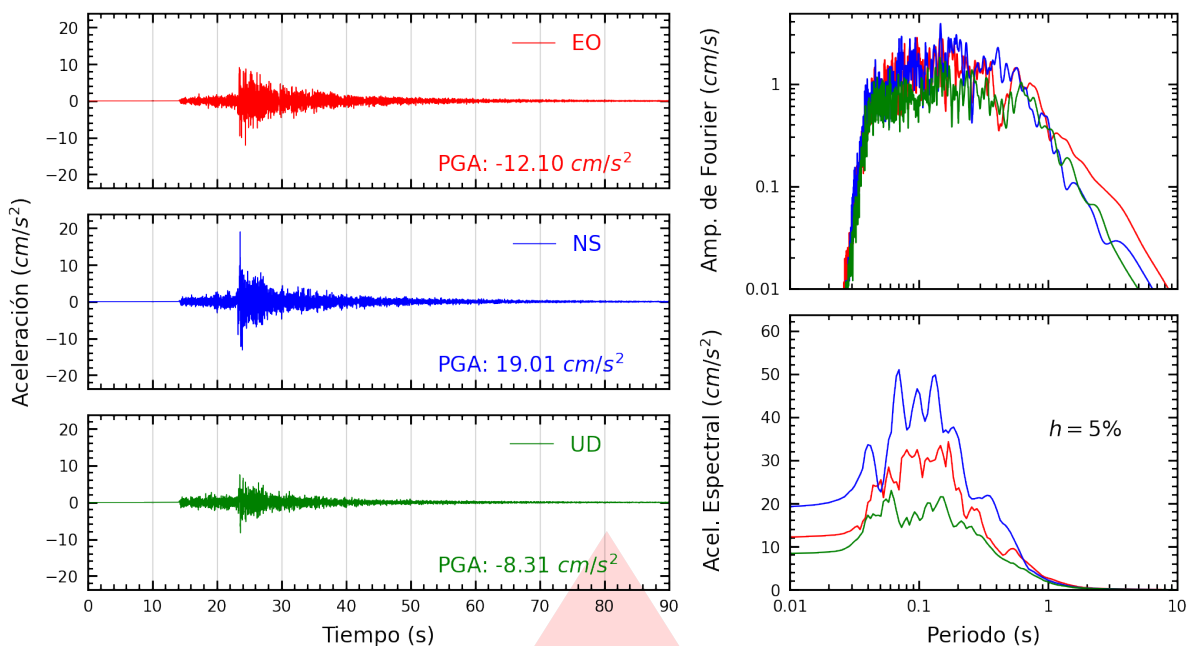
Figura A.1: Registros tiempo-historia, espectros de Fourier y de respuesta en las direcciones EO, NS y vertical de la estación UNSA2. Sismo de Quilca, Camaná - Arequipa del 2026-10-11, 08:43:01 (Hora local)
