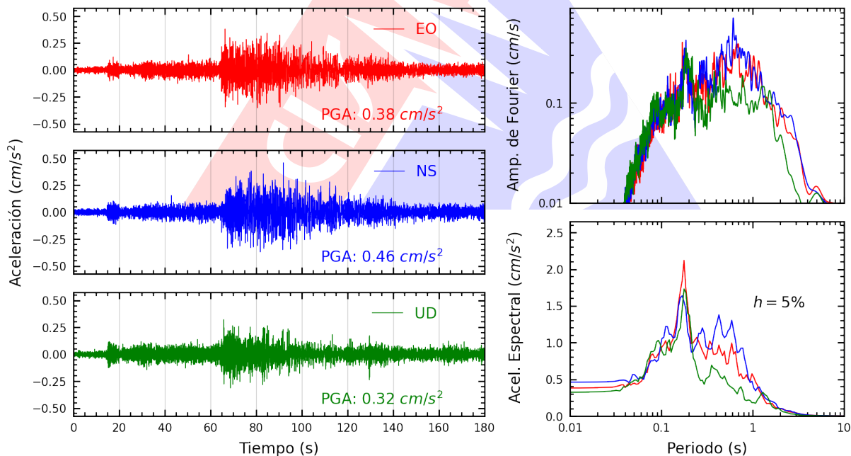
Figura A.6: Registros tiempo-historia, espectros de Fourier y de respuesta en las direcciones EO, NS y vertical de la estación UNICA. Sismo de Quilca, Camaná - Arequipa del 2026-10-11, 08:43:01 (Hora local)
