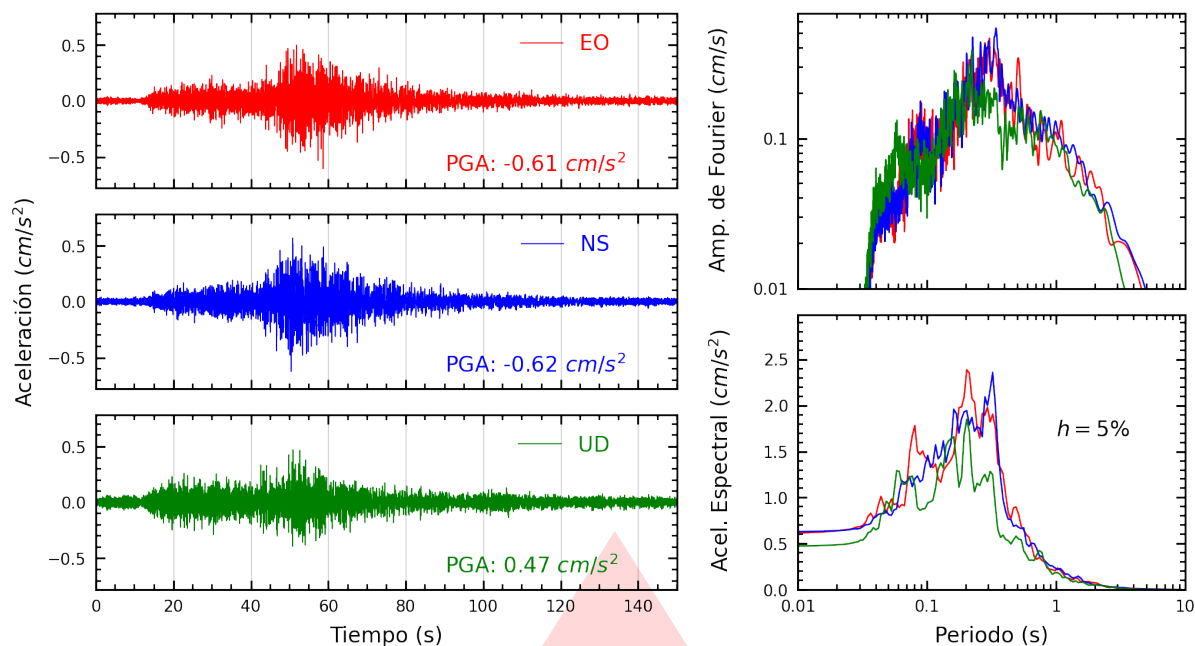
Figura A.5: Registros tiempo-historia, espectros de Fourier y de respuesta en las direcciones EO, NS y vertical de la estación UJBG2. Sismo de Quilca, Camaná - Arequipa del 2026-10-11, 08:43:01 (Hora local)
