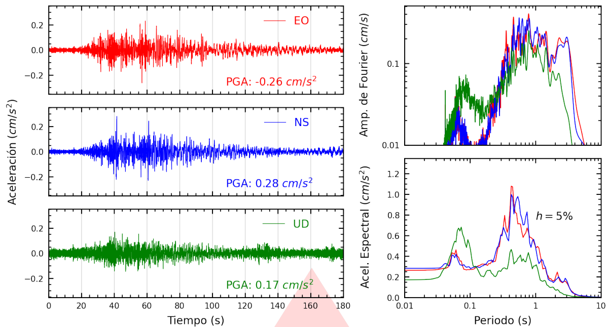
Figura A.7: Registros tiempo-historia, espectros de Fourier y de respuesta en las direcciones EO, NS y vertical de la estación UNAJ. Sismo de Quilca, Camaná - Arequipa del 2026-10-11, 08:43:01 (Hora local)
