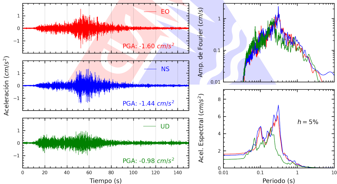
Figura A.2: Registros tiempo-historia, espectros de Fourier y de respuesta en las direcciones EO, NS y vertical de la estación SCTAC. Sismo de Quilca, Camaná - Arequipa del 2026-10-11, 08:43:01 (Hora local)
