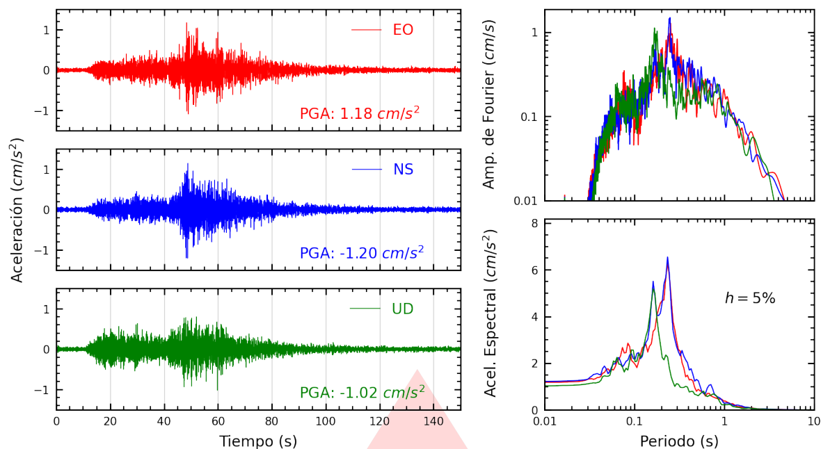
Figura A.3: Registros tiempo-historia, espectros de Fourier y de respuesta en las direcciones EO, NS y vertical de la estación UJBG4. Sismo de Quilca, Camaná - Arequipa del 2026-10-11, 08:43:01 (Hora local)
