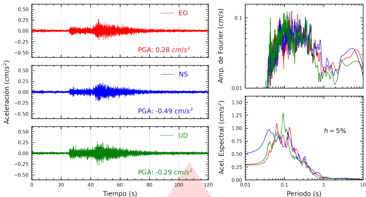
Figura A.33: Registros tiempo-historia, espectros de Fourier y de respuesta en las direcciones EO, NS y vertical de la estación BONDY. Sismo de Cañete, Cañete - Lima del 2026-10-12, 04:57:21 (Hora local)
