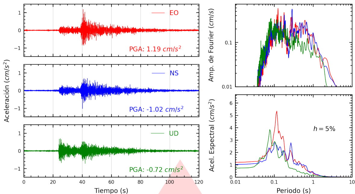
Figura A.13: Registros tiempo-historia, espectros de Fourier y de respuesta en las direcciones EO, NS y vertical de la estación UNICA. Sismo de Cañete, Cañete - Lima del 2026-10-12, 04:57:21 (Hora local)
