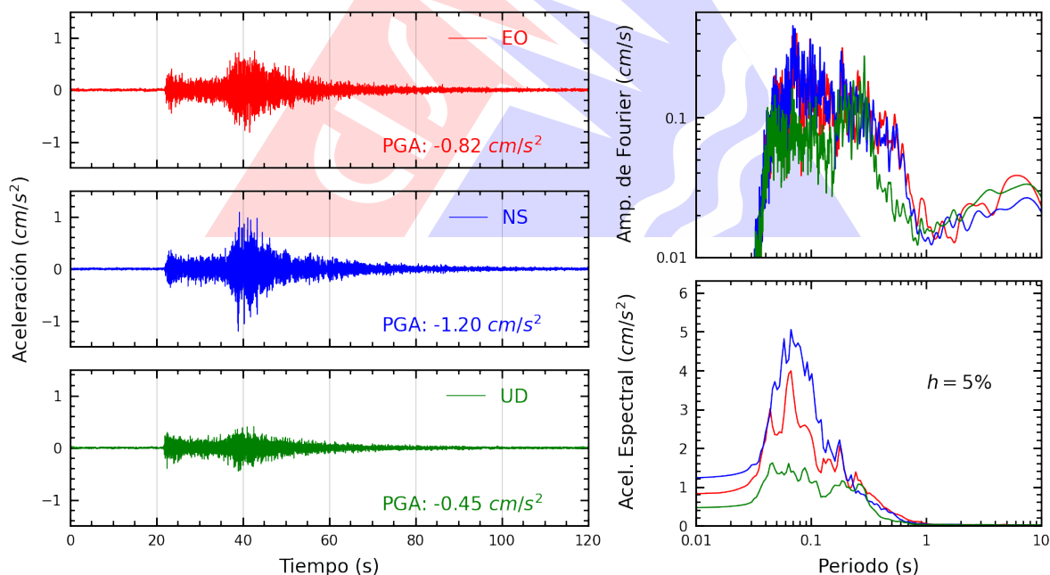
Figura A.12: Registros tiempo-historia, espectros de Fourier y de respuesta en las direcciones EO, NS y vertical de la estación UPCVI. Sismo de Cañete, Cañete - Lima del 2026-10-12, 04:57:21 (Hora local)
