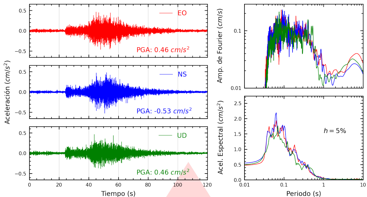
Figura A.29: Registros tiempo-historia, espectros de Fourier y de respuesta en las direcciones EO, NS y vertical de la estación IMCA. Sismo de Cañete, Cañete - Lima del 2026-10-12, 04:57:21 (Hora local)
