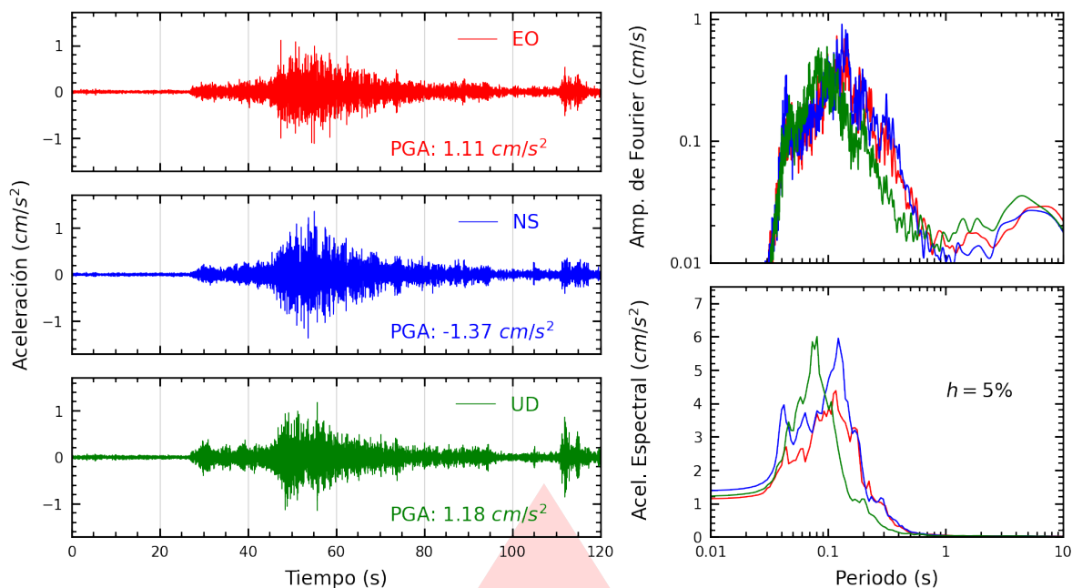
Figura A.11: Registros tiempo-historia, espectros de Fourier y de respuesta en las direcciones EO, NS y vertical de la estación CARAB. Sismo de Cañete, Cañete - Lima del 2026-10-12, 04:57:21 (Hora local)
