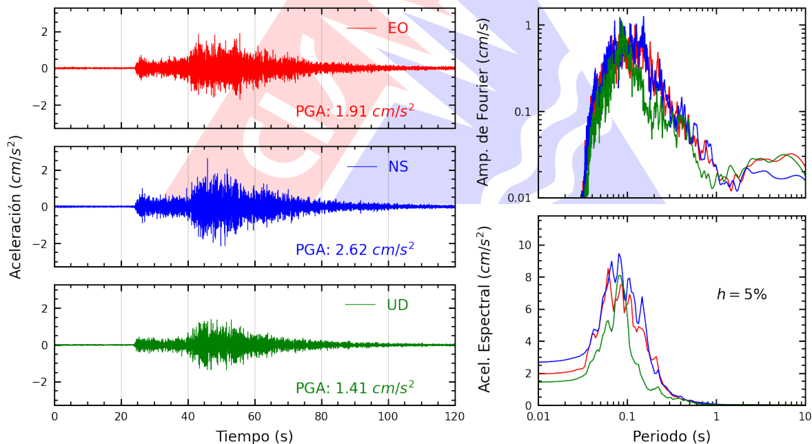
Figura A.2: Registros tiempo-historia, espectros de Fourier y de respuesta en las direcciones EO, NS y vertical de la estación USILM. Sismo de Cañete, Cañete - Lima del 2026-10-12, 04:57:21 (Hora local)
