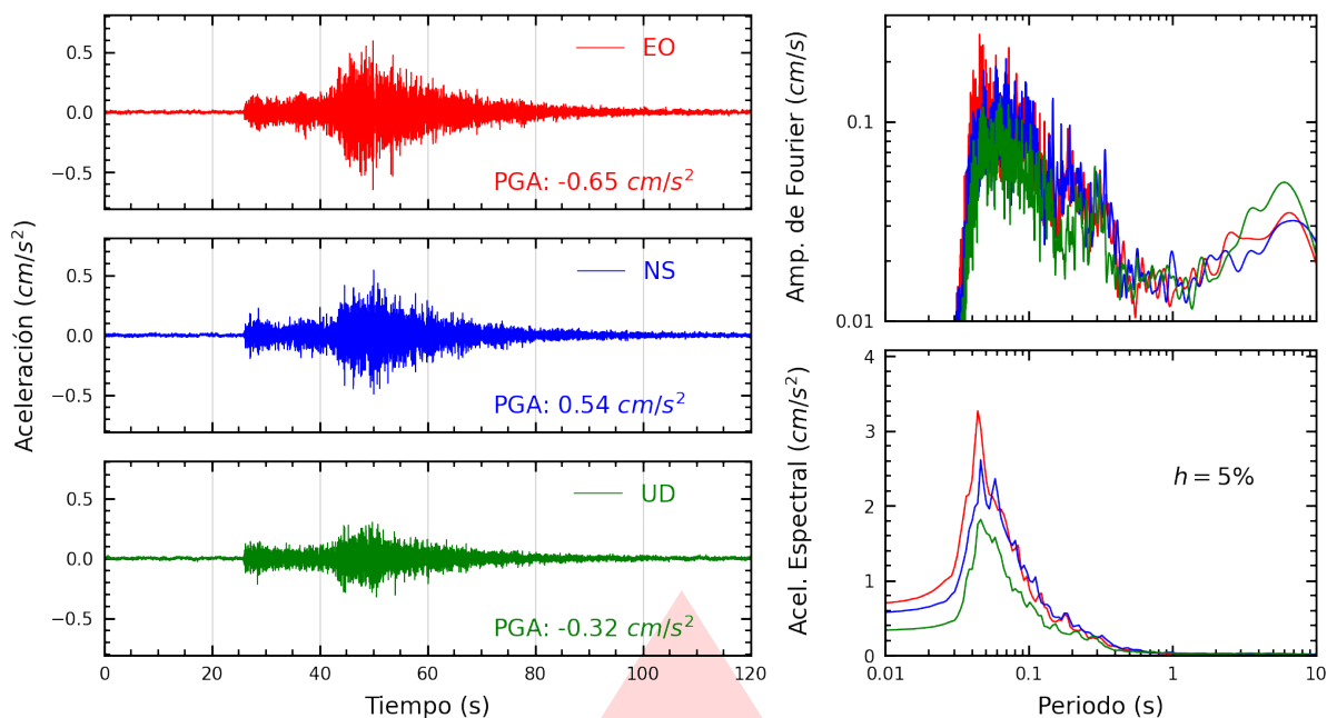
Figura A.21: Registros tiempo-historia, espectros de Fourier y de respuesta en las direcciones EO, NS y vertical de la estación UCSS. Sismo de Cañete, Cañete - Lima del 2026-10-12, 04:57:21 (Hora local)
