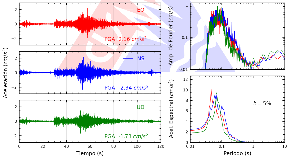
Figura A.4: Registros tiempo-historia, espectros de Fourier y de respuesta en las direcciones EO, NS y vertical de la estación SROSA. Sismo de Cañete, Cañete - Lima del 2026-10-12, 04:57:21 (Hora local)
