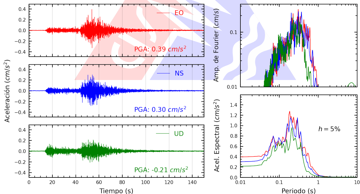
Figura A.34: Registros tiempo-historia, espectros de Fourier y de respuesta en las direcciones EO, NS y vertical de la estación CARAL. Sismo de Cañete, Cañete - Lima del 2026-10-12, 04:57:21 (Hora local)
