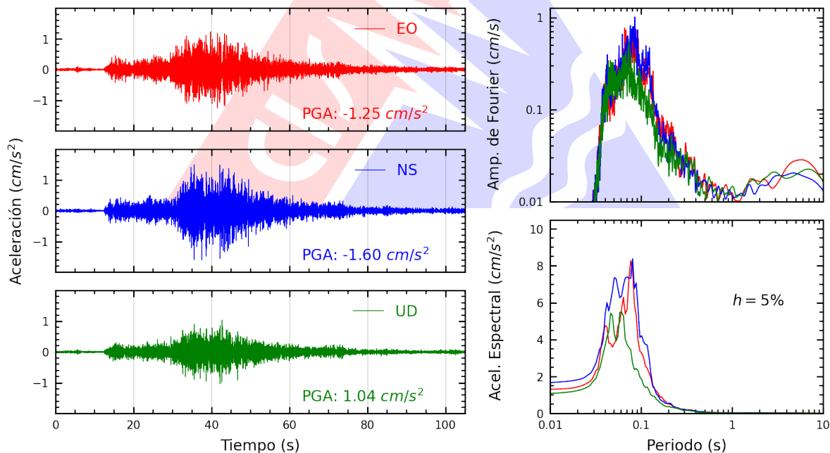
Figura A.6: Registros tiempo-historia, espectros de Fourier y de respuesta en las direcciones EO, NS y vertical de la estación JOSEO. Sismo de Cañete, Cañete - Lima del 2026-10-12, 04:57:21 (Hora local)
