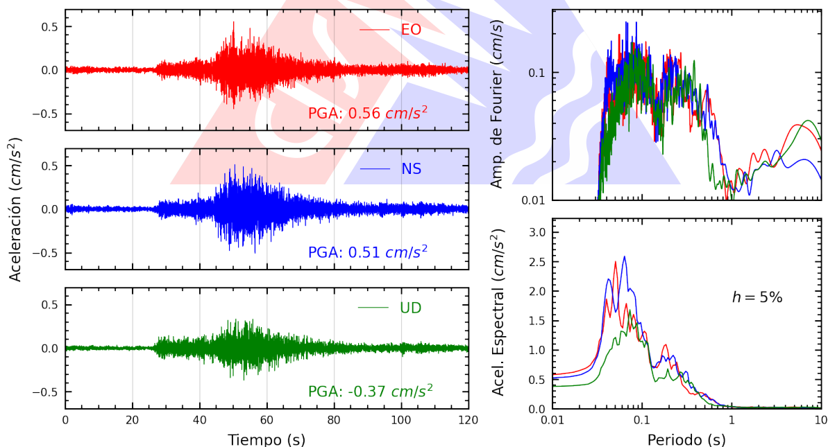
Figura A.26: Registros tiempo-historia, espectros de Fourier y de respuesta en las direcciones EO, NS y vertical de la estación COMAS. Sismo de Cañete, Cañete - Lima del 2026-10-12, 04:57:21 (Hora local)
