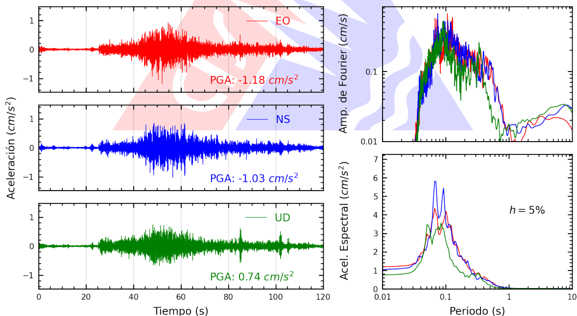
Figura A.14: Registros tiempo-historia, espectros de Fourier y de respuesta en las direcciones EO, NS y vertical de la estación SJLSV. Sismo de Cañete, Cañete - Lima del 2026-10-12, 04:57:21 (Hora local)
