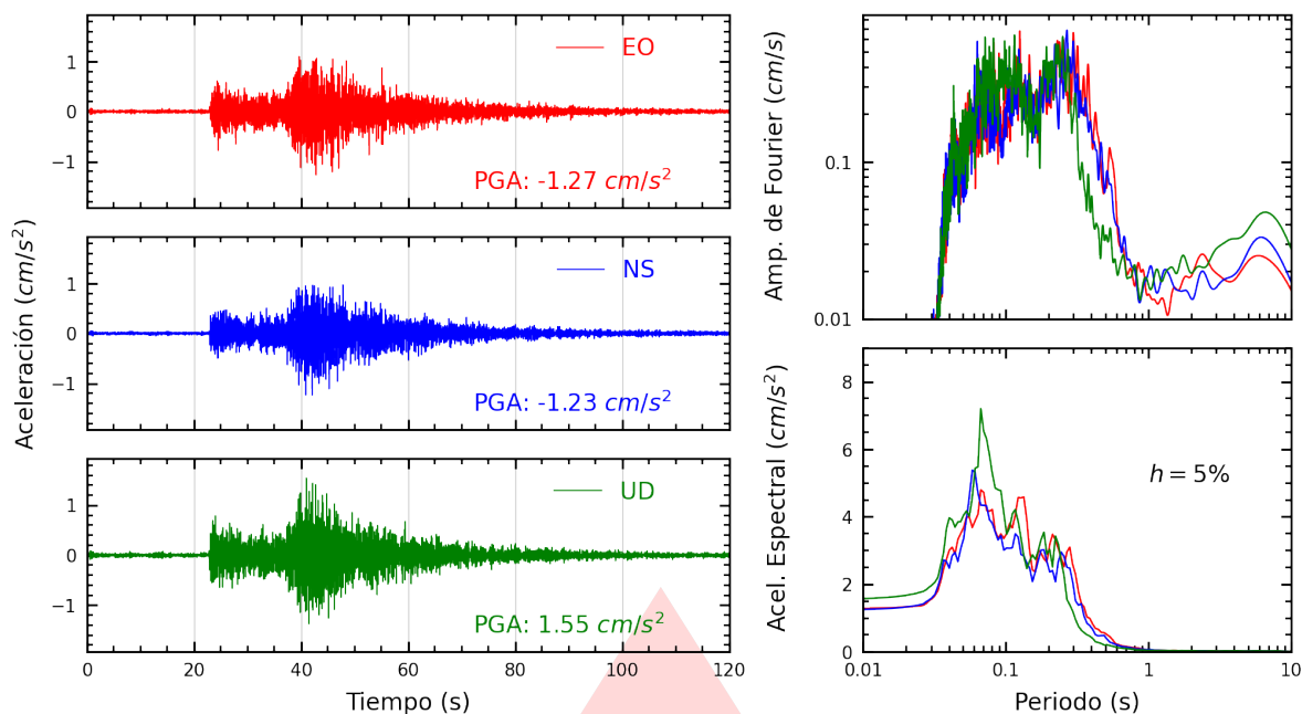
Figura A.7: Registros tiempo-historia, espectros de Fourier y de respuesta en las direcciones EO, NS y vertical de la estación SOVES. Sismo de Cañete, Cañete - Lima del 2026-10-12, 04:57:21 (Hora local)
