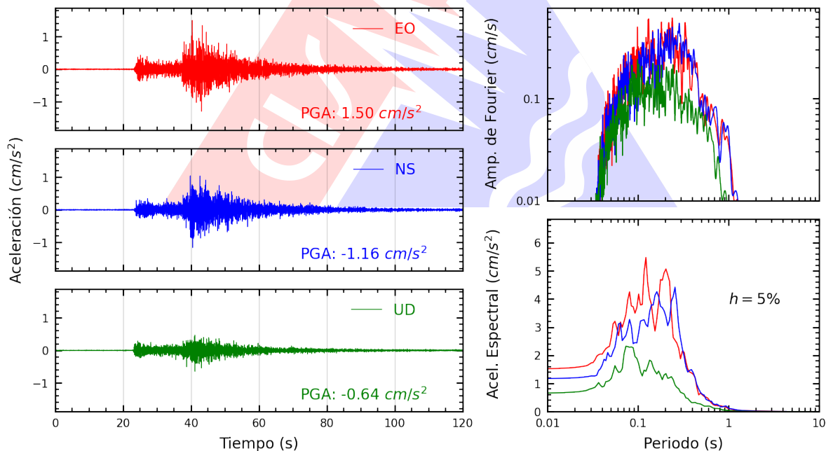
Figura A.8: Registros tiempo-historia, espectros de Fourier y de respuesta en las direcciones EO, NS y vertical de la estación BRISA. Sismo de Cañete, Cañete - Lima del 2026-10-12, 04:57:21 (Hora local)
