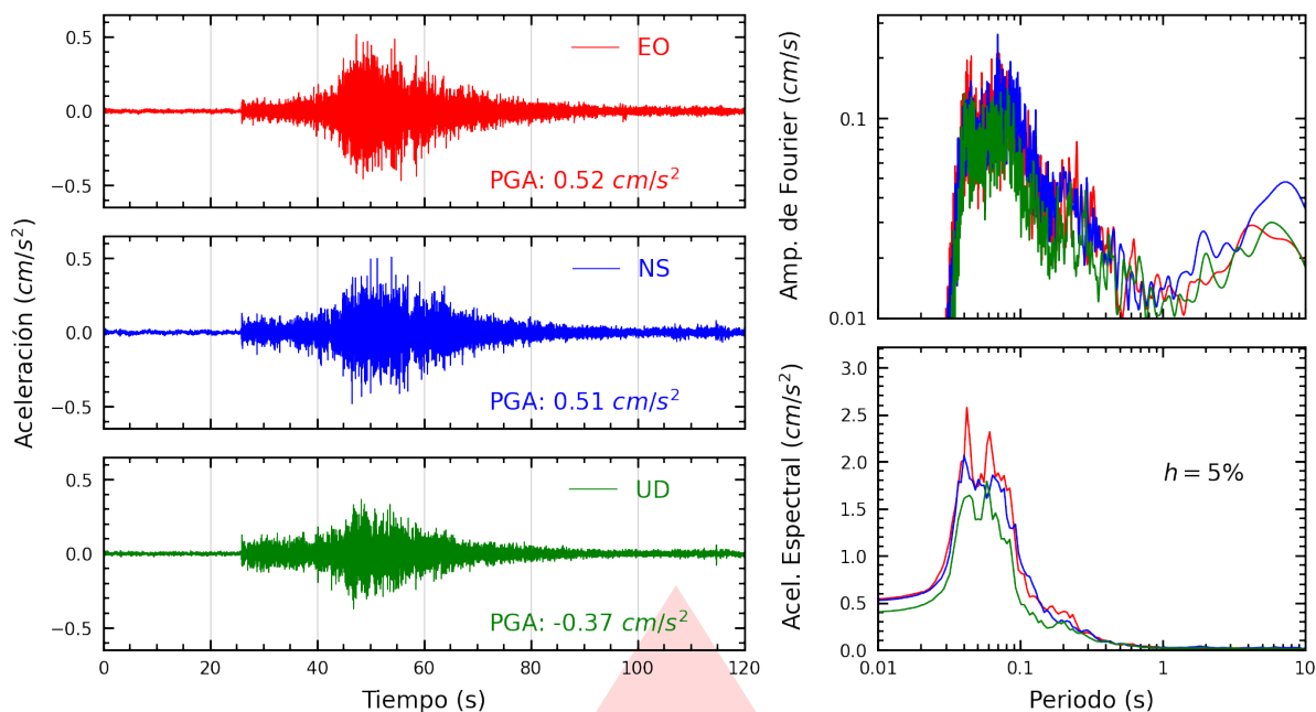
Figura A.31: Registros tiempo-historia, espectros de Fourier y de respuesta en las direcciones EO, NS y vertical de la estación SJLCE. Sismo de Cañete, Cañete - Lima del 2026-10-12, 04:57:21 (Hora local)
