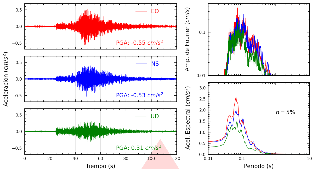
Figura A.27: Registros tiempo-historia, espectros de Fourier y de respuesta en las direcciones EO, NS y vertical de la estación ATARJ. Sismo de Cañete, Cañete - Lima del 2026-10-12, 04:57:21 (Hora local)
