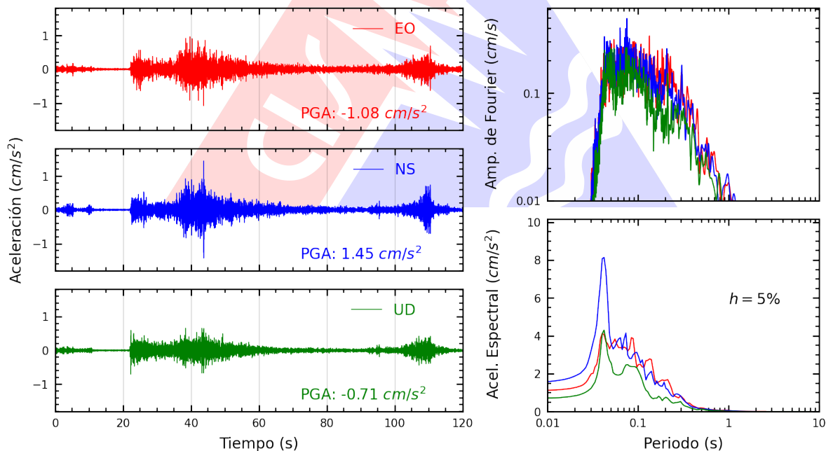
Figura A.10: Registros tiempo-historia, espectros de Fourier y de respuesta en las direcciones EO, NS y vertical de la estación PACHA. Sismo de Cañete, Cañete - Lima del 2026-10-12, 04:57:21 (Hora local)
