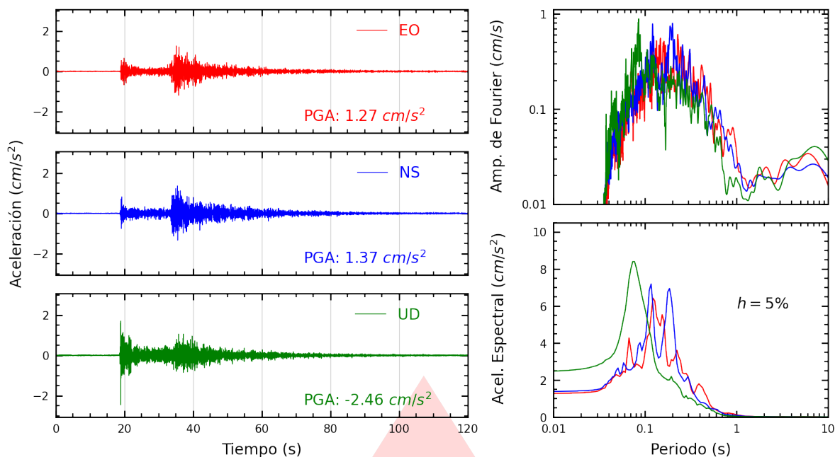
Figura A.3: Registros tiempo-historia, espectros de Fourier y de respuesta en las direcciones EO, NS y vertical de la estación SOCHO. Sismo de Cañete, Cañete - Lima del 2026-10-12, 04:57:21 (Hora local)
