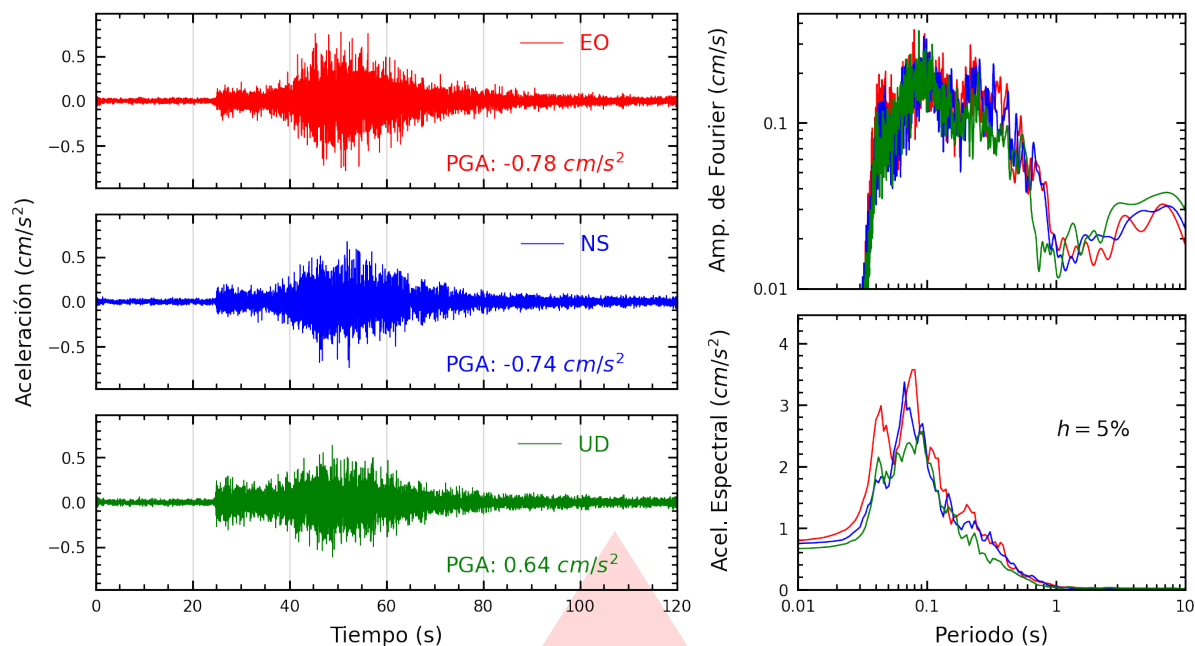
Figura A.19: Registros tiempo-historia, espectros de Fourier y de respuesta en las direcciones EO, NS y vertical de la estación UCVAT. Sismo de Cañete, Cañete - Lima del 2026-10-12, 04:57:21 (Hora local)
