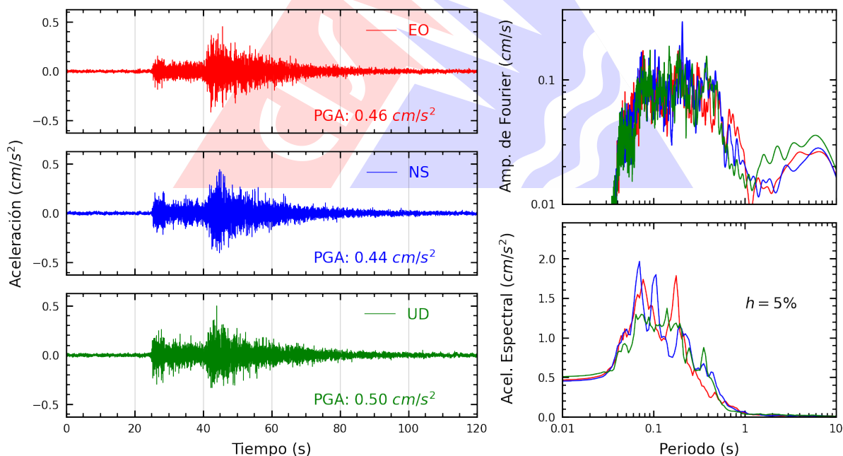
Figura A.32: Registros tiempo-historia, espectros de Fourier y de respuesta en las direcciones EO, NS y vertical de la estación UNFV. Sismo de Cañete, Cañete - Lima del 2026-10-12, 04:57:21 (Hora local)
