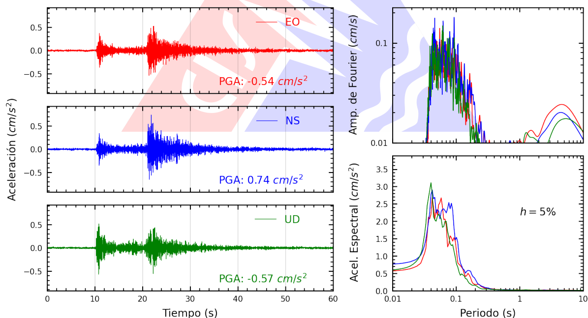
Figura A.22: Registros tiempo-historia, espectros de Fourier y de respuesta en las direcciones EO, NS y vertical de la estación SERVI. Sismo de Chosica, Lima - Lima del 2026-10-14, 20:16:04 (Hora local)
