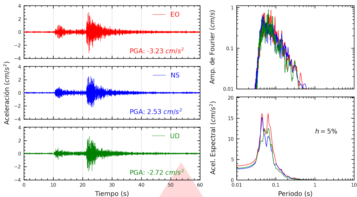
Figura A.3: Registros tiempo-historia, espectros de Fourier y de respuesta en las direcciones EO, NS y vertical de la estación UNTEL. Sismo de Chosica, Lima - Lima del 2026-10-14, 20:16:04 (Hora local)
