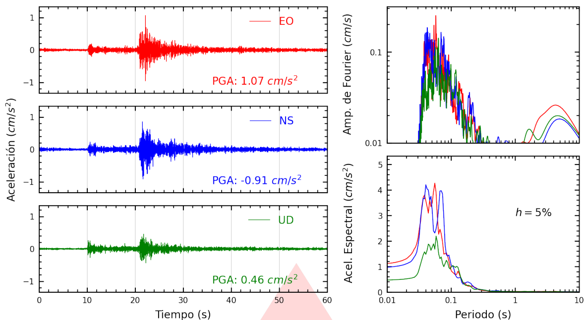
Figura A.17: Registros tiempo-historia, espectros de Fourier y de respuesta en las direcciones EO, NS y vertical de la estación COMAS. Sismo de Chosica, Lima - Lima del 2026-10-14, 20:16:04 (Hora local)
