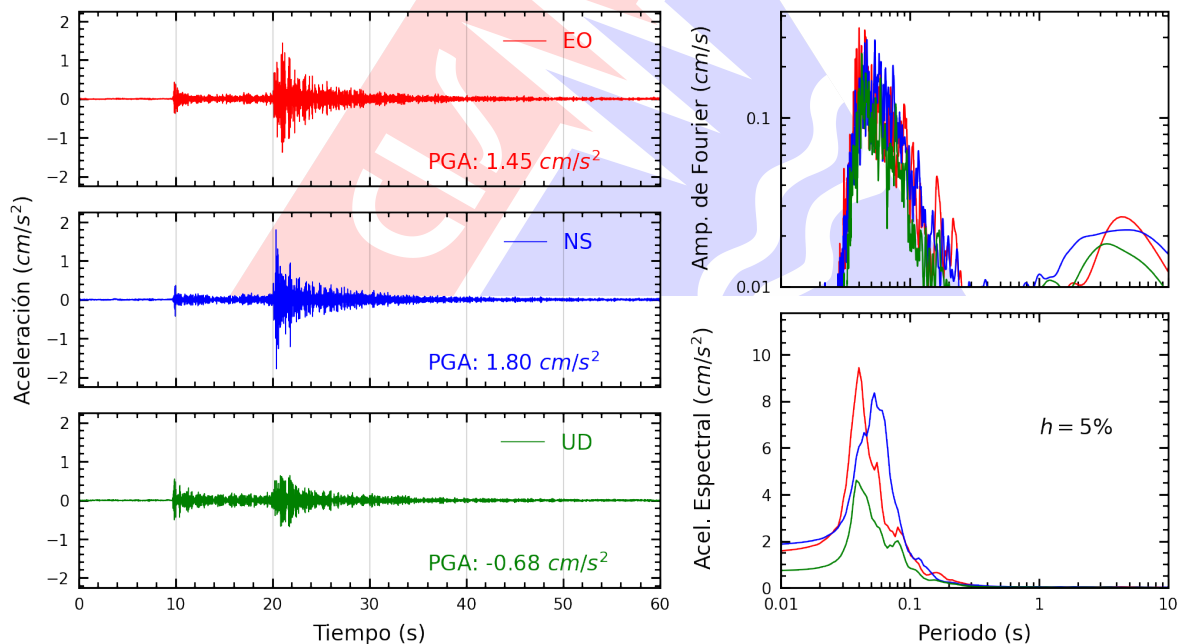
Figura A.10: Registros tiempo-historia, espectros de Fourier y de respuesta en las direcciones EO, NS y vertical de la estación SJLCE. Sismo de Chosica, Lima - Lima del 2026-10-14, 20:16:04 (Hora local)
