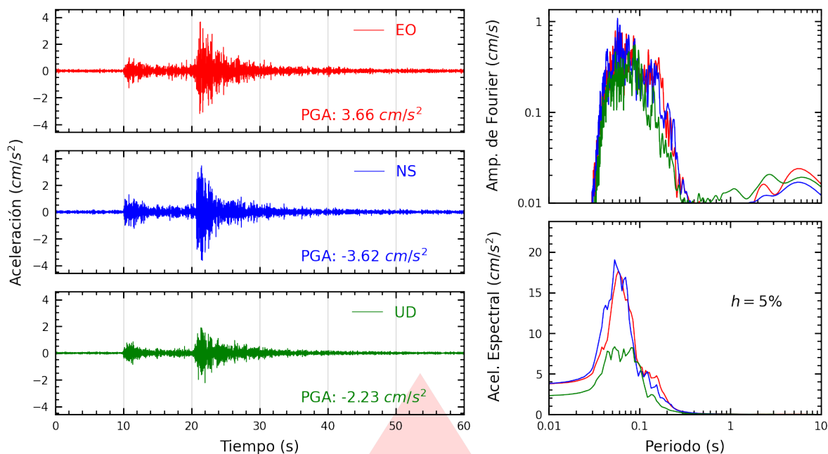
Figura A.1: Registros tiempo-historia, espectros de Fourier y de respuesta en las direcciones EO, NS y vertical de la estación USILM. Sismo de Chosica, Lima - Lima del 2026-10-14, 20:16:04 (Hora local)
