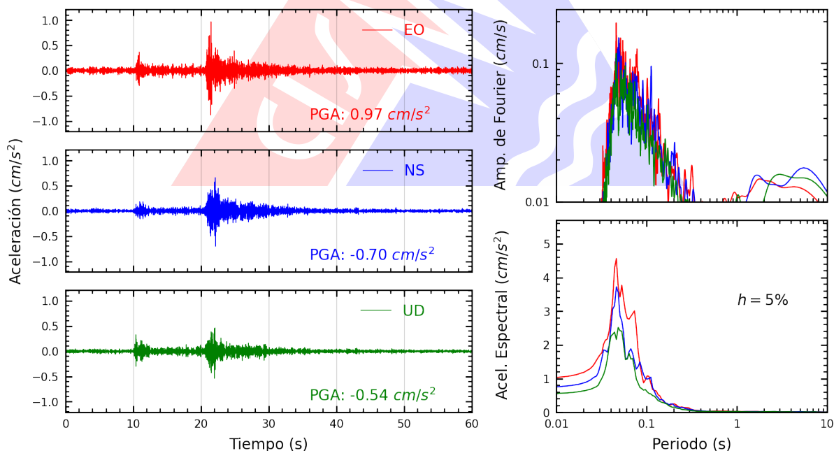
Figura A.18: Registros tiempo-historia, espectros de Fourier y de respuesta en las direcciones EO, NS y vertical de la estación INICT. Sismo de Chosica, Lima - Lima del 2026-10-14, 20:16:04 (Hora local)
