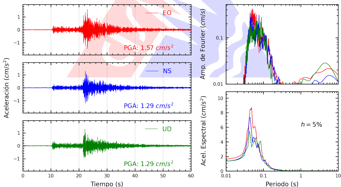
Figura A.14: Registros tiempo-historia, espectros de Fourier y de respuesta en las direcciones EO, NS y vertical de la estación AMORE. Sismo de Chosica, Lima - Lima del 2026-10-14, 20:16:04 (Hora local)
