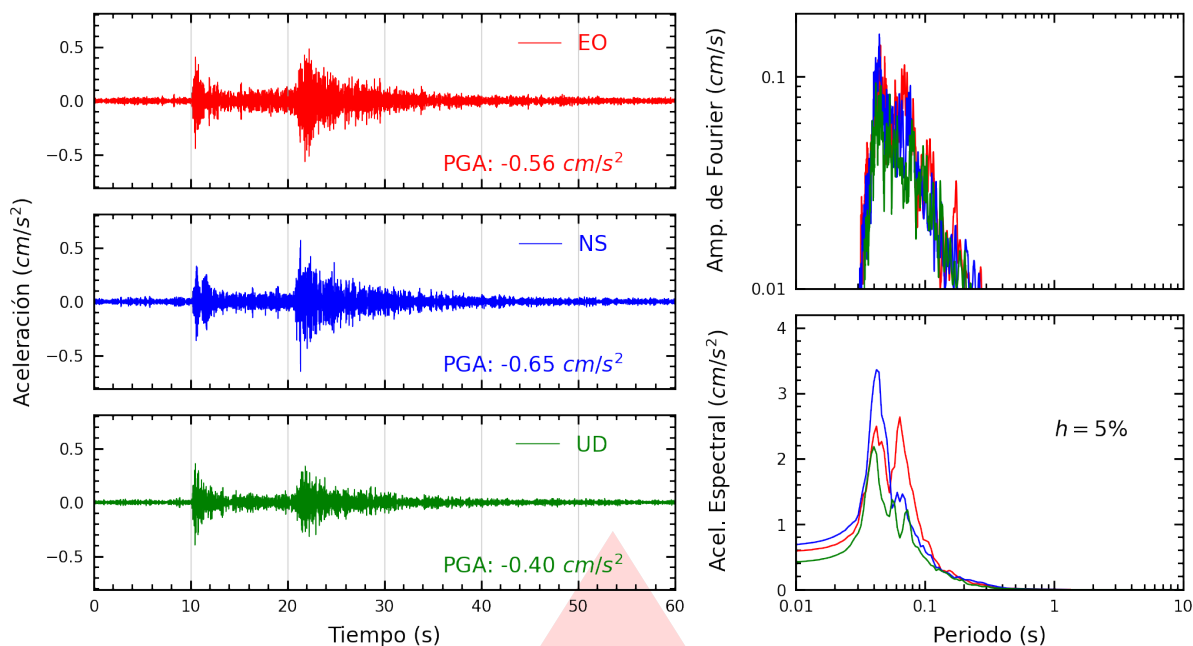
Figura A.23: Registros tiempo-historia, espectros de Fourier y de respuesta en las direcciones EO, NS y vertical de la estación BORJA. Sismo de Chosica, Lima - Lima del 2026-10-14, 20:16:04 (Hora local)
