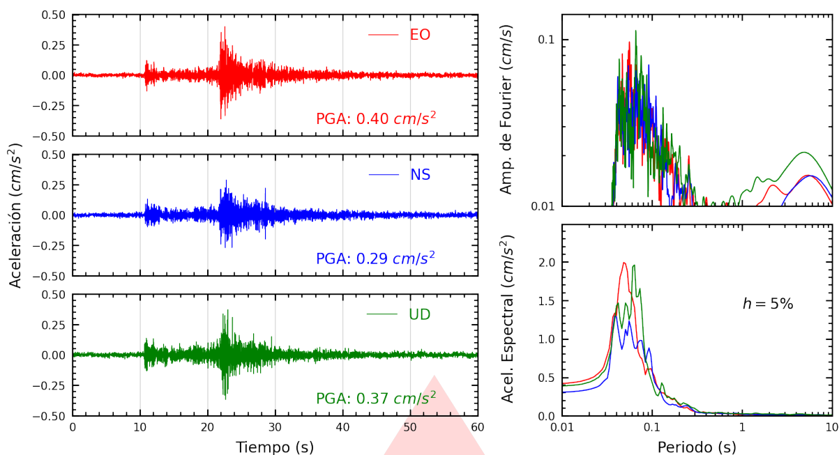
Figura A.25: Registros tiempo-historia, espectros de Fourier y de respuesta en las direcciones EO, NS y vertical de la estación UNFV. Sismo de Chosica, Lima - Lima del 2026-10-14, 20:16:04 (Hora local)
