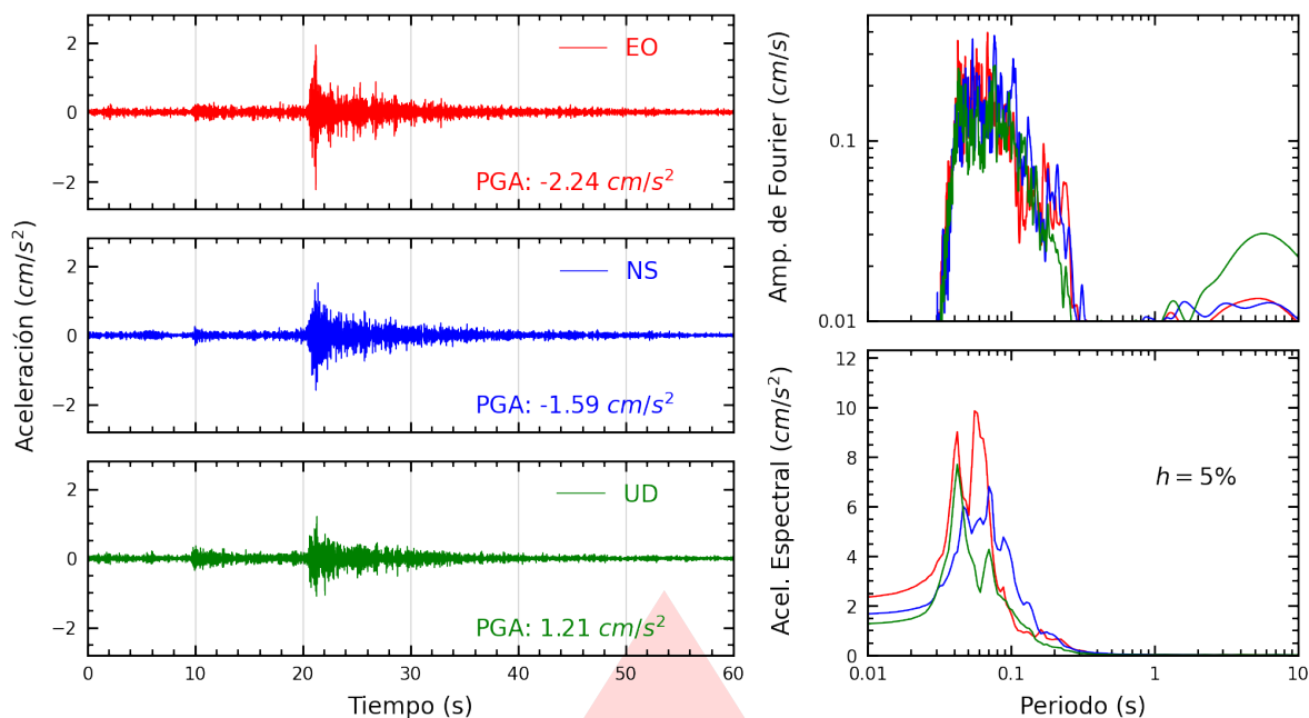
Figura A.7: Registros tiempo-historia, espectros de Fourier y de respuesta en las direcciones EO, NS y vertical de la estación INDEP. Sismo de Chosica, Lima - Lima del 2026-10-14, 20:16:04 (Hora local)
