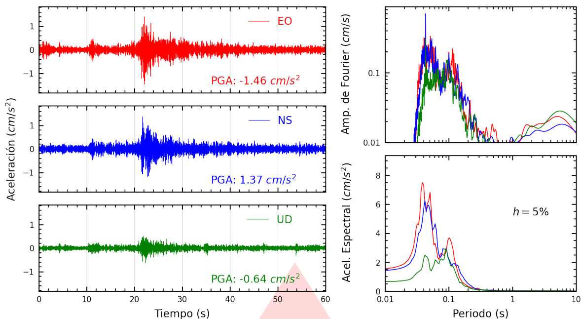
Figura A.15: Registros tiempo-historia, espectros de Fourier y de respuesta en las direcciones EO, NS y vertical de la estación OLIVO. Sismo de Chosica, Lima - Lima del 2026-10-14, 20:16:04 (Hora local)
