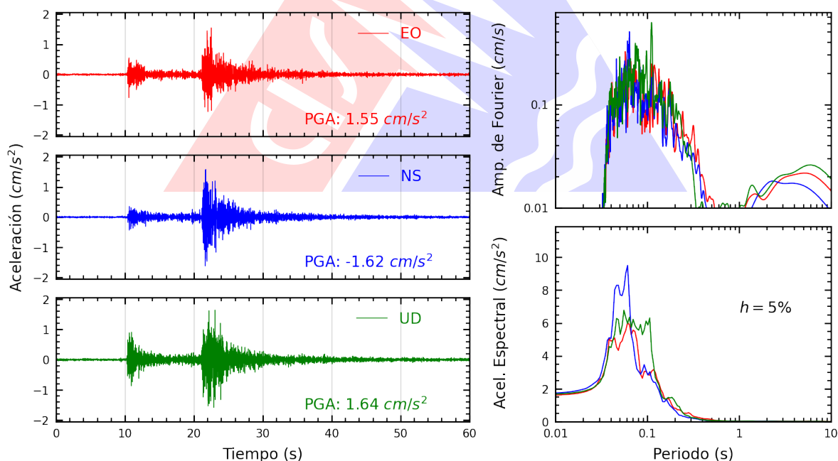
Figura A.12: Registros tiempo-historia, espectros de Fourier y de respuesta en las direcciones EO, NS y vertical de la estación SOVES. Sismo de Chosica, Lima - Lima del 2026-10-14, 20:16:04 (Hora local)
