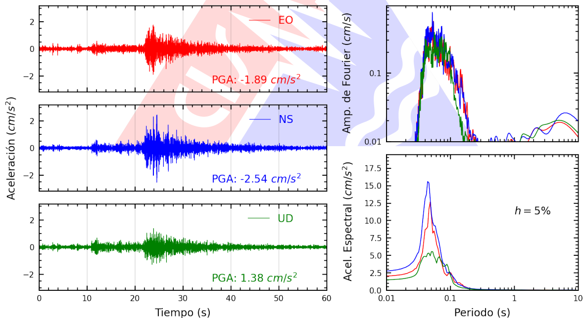
Figura A.6: Registros tiempo-historia, espectros de Fourier y de respuesta en las direcciones EO, NS y vertical de la estación SROSA. Sismo de Chosica, Lima - Lima del 2026-10-14, 20:16:04 (Hora local)
