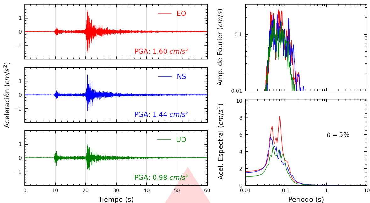
Figura A.13: Registros tiempo-historia, espectros de Fourier y de respuesta en las direcciones EO, NS y vertical de la estación ATARJ. Sismo de Chosica, Lima - Lima del 2026-10-14, 20:16:04 (Hora local)
