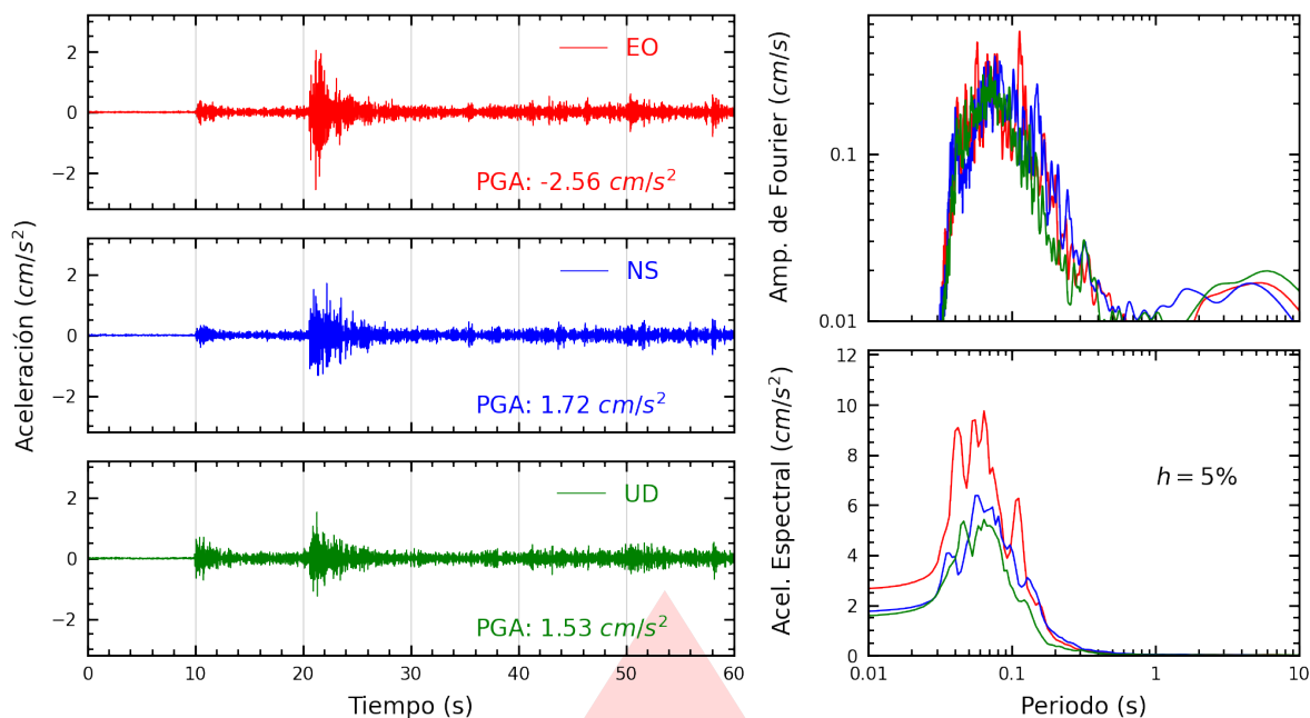
Figura A.5: Registros tiempo-historia, espectros de Fourier y de respuesta en las direcciones EO, NS y vertical de la estación SJLSV. Sismo de Chosica, Lima - Lima del 2026-10-14, 20:16:04 (Hora local)
