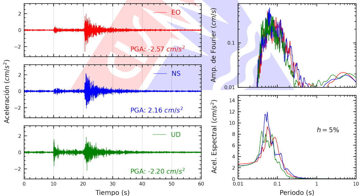
Figura A.4: Registros tiempo-historia, espectros de Fourier y de respuesta en las direcciones EO, NS y vertical de la estación SJLSC. Sismo de Chosica, Lima - Lima del 2026-10-14, 20:16:04 (Hora local)
