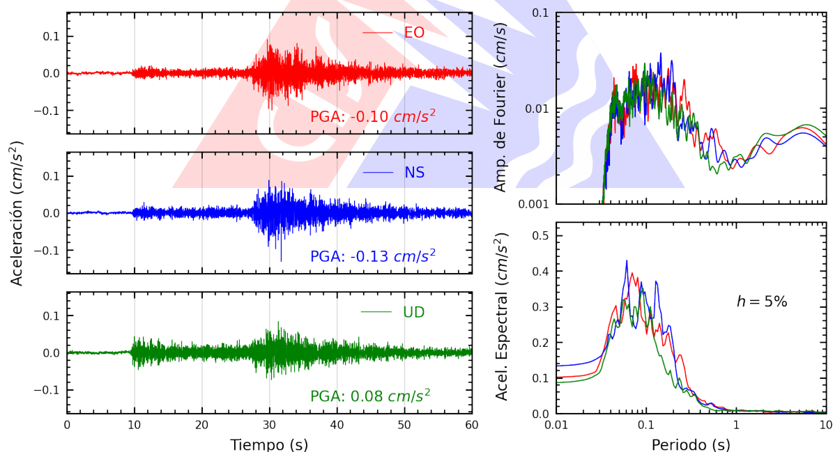
Figura A.26: Registros tiempo-historia, espectros de Fourier y de respuesta en las direcciones EO, NS y vertical de la estación CARAL. Sismo de Chosica, Lima - Lima del 2026-10-14, 20:16:04 (Hora local)
