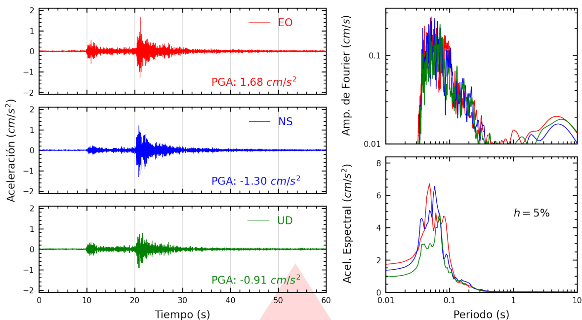
Figura A.11: Registros tiempo-historia, espectros de Fourier y de respuesta en las direcciones EO, NS y vertical de la estación IMCA. Sismo de Chosica, Lima - Lima del 2026-10-14, 20:16:04 (Hora local)
