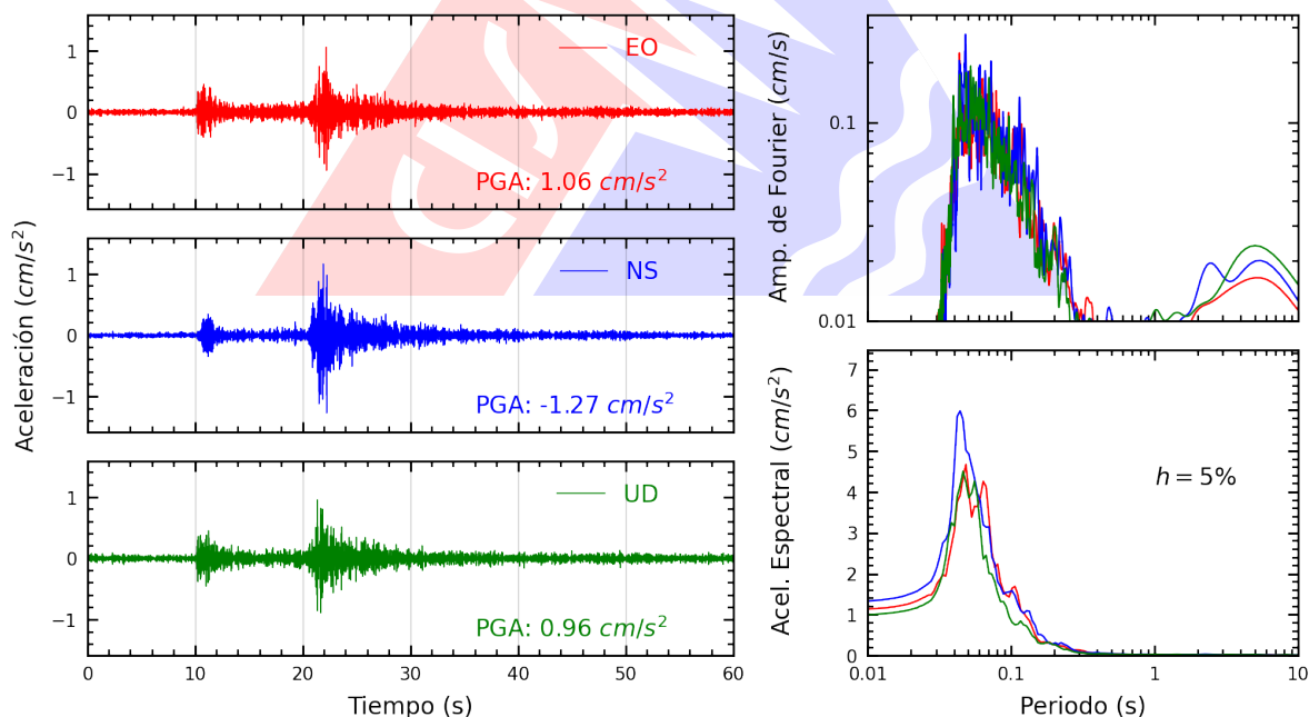
Figura A.16: Registros tiempo-historia, espectros de Fourier y de respuesta en las direcciones EO, NS y vertical de la estación URPPE. Sismo de Chosica, Lima - Lima del 2026-10-14, 20:16:04 (Hora local)
