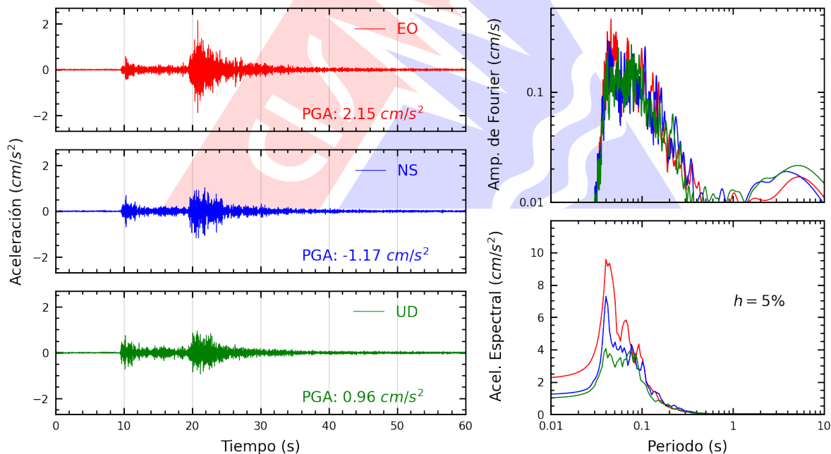
Figura A.8: Registros tiempo-historia, espectros de Fourier y de respuesta en las direcciones EO, NS y vertical de la estación UCVAT. Sismo de Chosica, Lima - Lima del 2026-10-14, 20:16:04 (Hora local)
