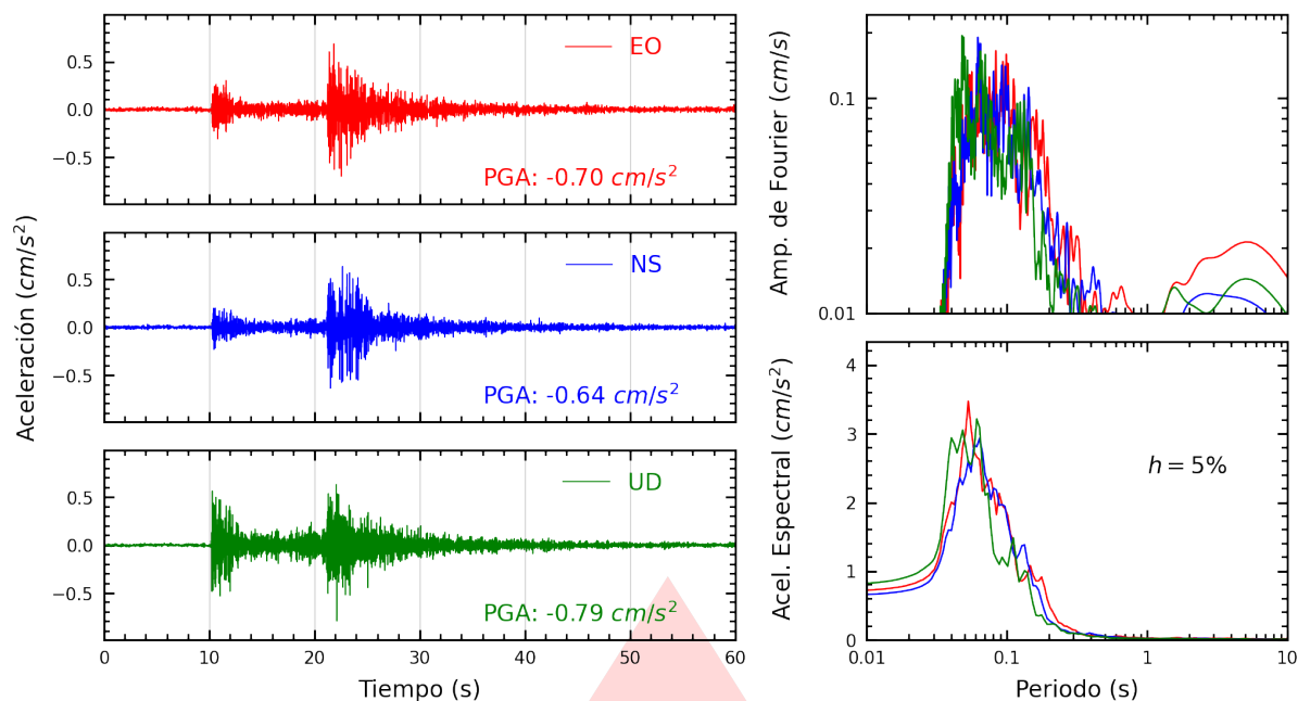
Figura A.21: Registros tiempo-historia, espectros de Fourier y de respuesta en las direcciones EO, NS y vertical de la estación USILP. Sismo de Chosica, Lima - Lima del 2026-10-14, 20:16:04 (Hora local)
