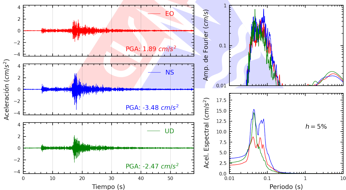
Figura A.2: Registros tiempo-historia, espectros de Fourier y de respuesta en las direcciones EO, NS y vertical de la estación JOSEO. Sismo de Chosica, Lima - Lima del 2026-10-14, 20:16:04 (Hora local)
