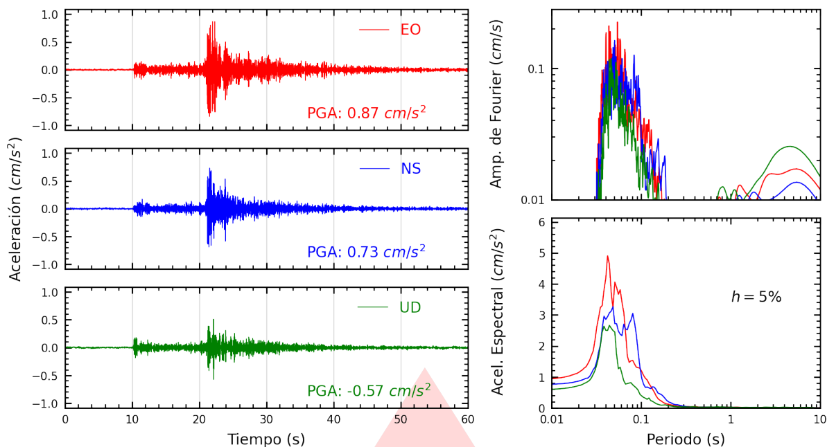
Figura A.19: Registros tiempo-historia, espectros de Fourier y de respuesta en las direcciones EO, NS y vertical de la estación UCSS. Sismo de Chosica, Lima - Lima del 2026-10-14, 20:16:04 (Hora local)
