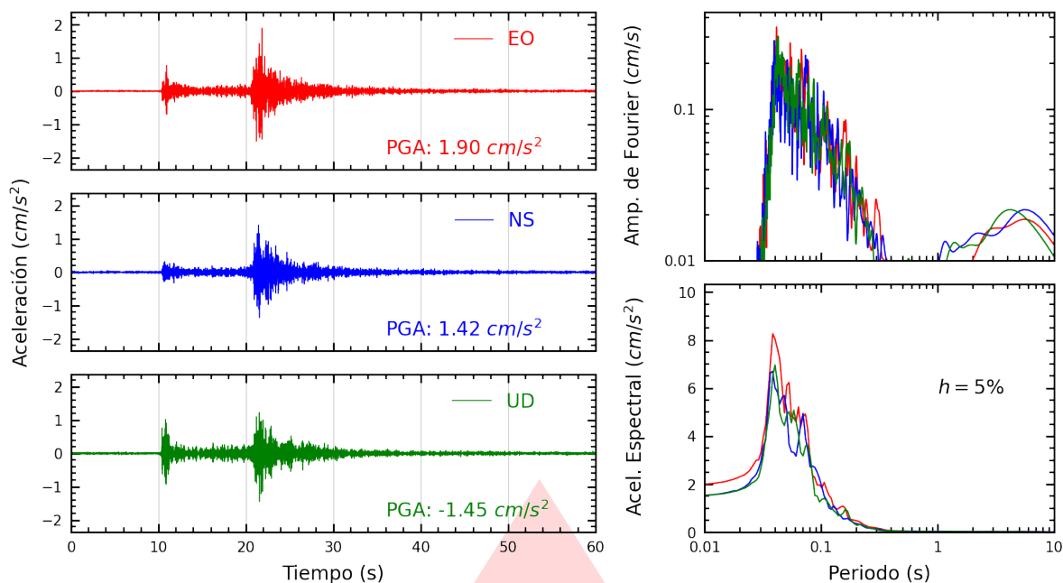
Figura A.9: Registros tiempo-historia, espectros de Fourier y de respuesta en las direcciones EO, NS y vertical de la estación USMP. Sismo de Chosica, Lima - Lima del 2026-10-14, 20:16:04 (Hora local)
