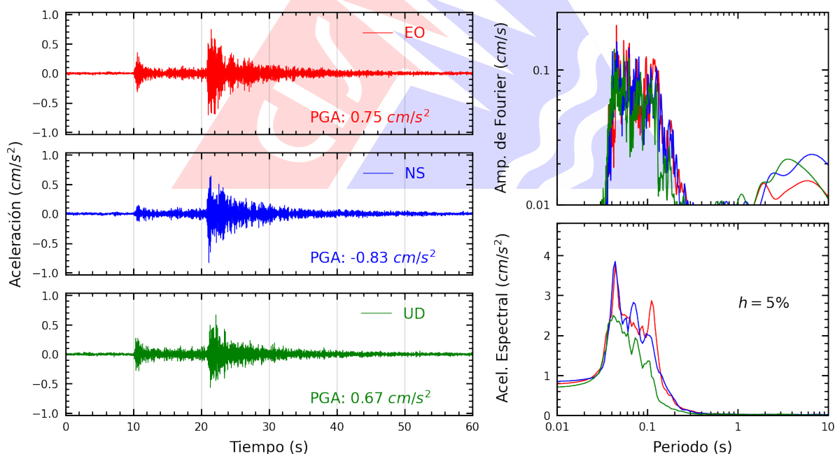
Figura A.20: Registros tiempo-historia, espectros de Fourier y de respuesta en las direcciones EO, NS y vertical de la estación JALVA. Sismo de Chosica, Lima - Lima del 2026-10-14, 20:16:04 (Hora local)
