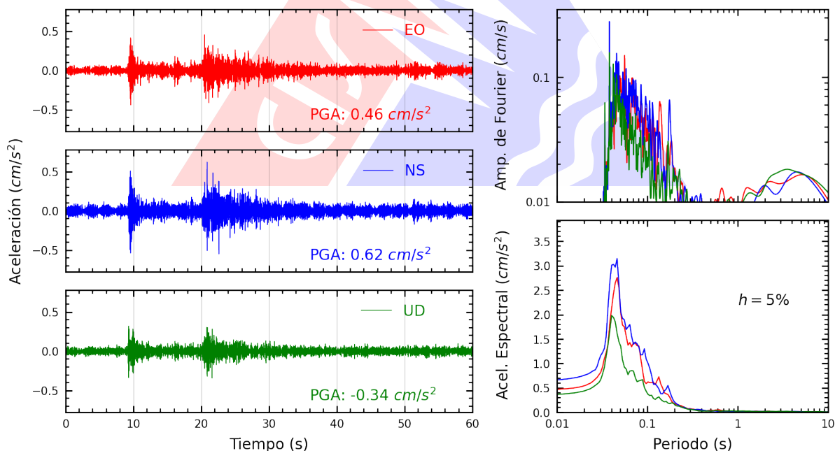
Figura A.24: Registros tiempo-historia, espectros de Fourier y de respuesta en las direcciones EO, NS y vertical de la estación UPCVI. Sismo de Chosica, Lima - Lima del 2026-10-14, 20:16:04 (Hora local)
