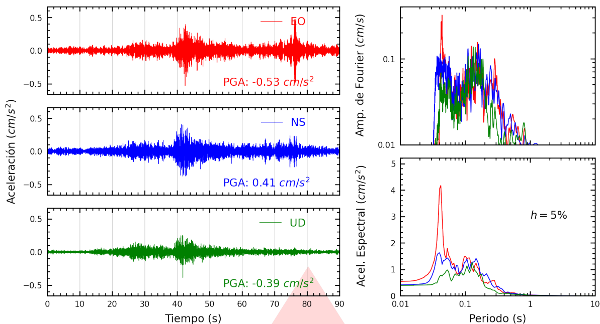
Figura A.1: Registros tiempo-historia, espectros de Fourier y de respuesta en las direcciones EO, NS y vertical de la estación UPTAC. Sismo de Conduriri, El Collao - Puno del 2026-10-30, 17:46:56 (Hora local)
