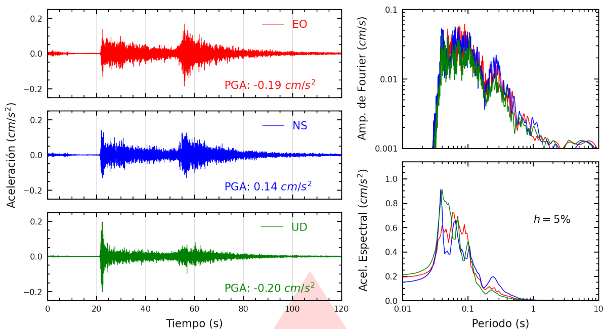
Figura A.5: Registros tiempo-historia, espectros de Fourier y de respuesta en las direcciones EO, NS y vertical de la estación UNSA2. Sismo de Conduriri, El Collao - Puno del 2026-10-30, 17:46:56 (Hora local)
