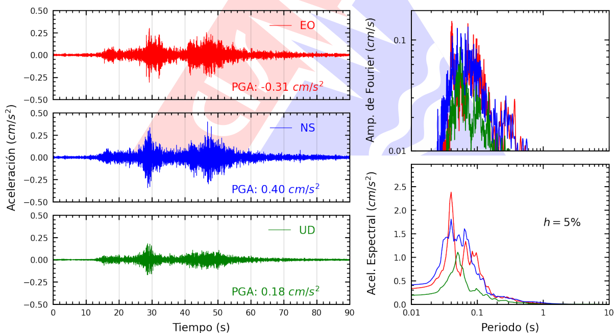
Figura A.4: Registros tiempo-historia, espectros de Fourier y de respuesta en las direcciones EO, NS y vertical de la estación UNAM. Sismo de Conduriri, El Collao - Puno del 2026-10-30, 17:46:56 (Hora local)
