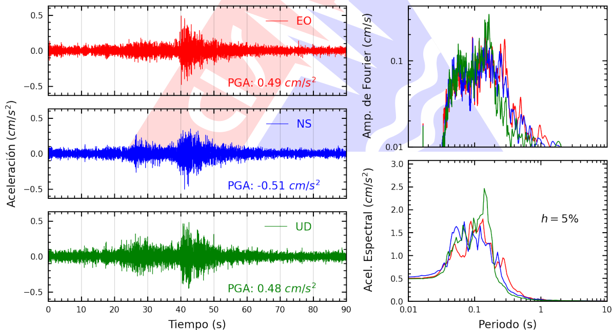
Figura A.2: Registros tiempo-historia, espectros de Fourier y de respuesta en las direcciones EO, NS y vertical de la estación UJB4. Sismo de Conduriri, El Collao - Puno del 2026-10-30, 17:46:56 (Hora local)
